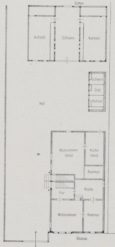
Abb. 51 b. Erdgeschoßgrundriß.
