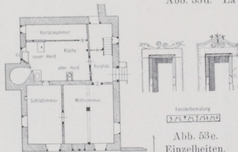
Abb. 53b. Erdgeschoß.
