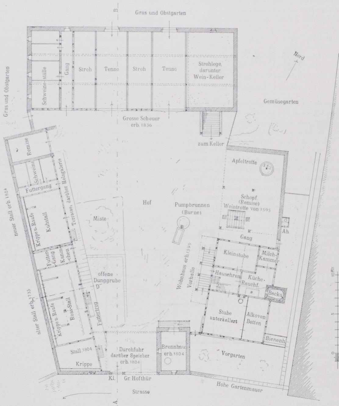
Abb. 30. Grundriß der Hofanlage des Bauernhofes Jacob in Büsweiler (Unter-Elsaß).
