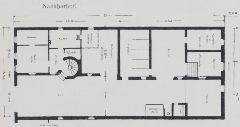
Abb. 1. Erdgeschoß-Grundriß.
