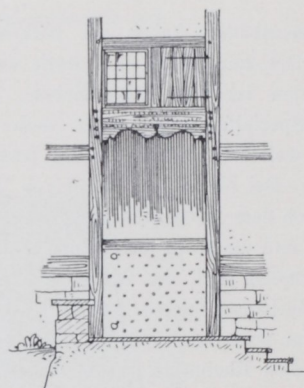
Abb. 5. Türe bei a in Abb. 1.
