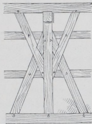
Abb. 17 und 18. Typen von Verstrebung und Gefachfüllung.
