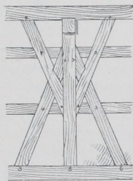
Abb. 17 und 18. Typen von Verstrebung und Gefachfüllung.
