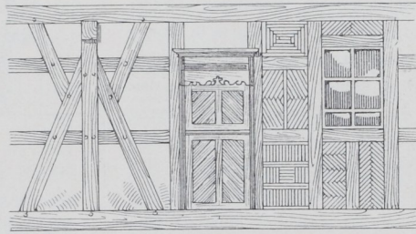
Abb. 17 und 18. Typen von Verstrebung und Gefachfüllung.
