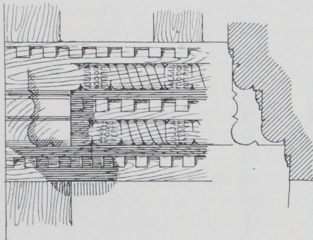
Abb. 13. Gebälk aus Wahlwinkel Nr. 19, bei Waltershausen.
