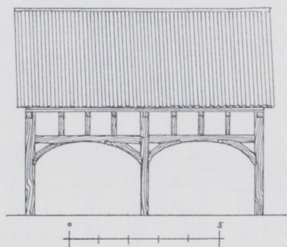
Abb. 4. Schuppen in Ilmenau.
