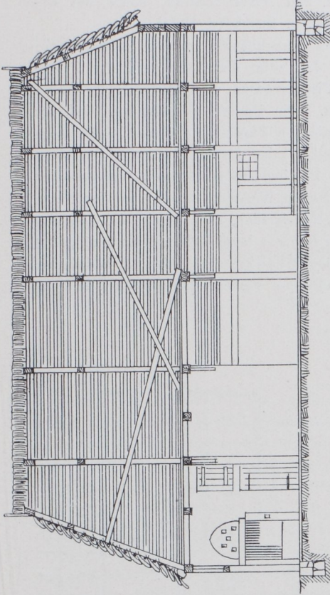
Abb. 2. Längenschnitt.
