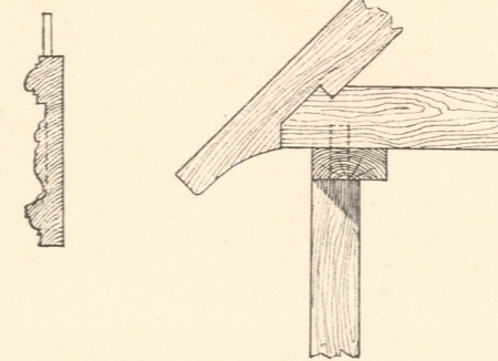
Abb. 8. Verbindung von Wandstiel Rähm, Balken u. Sparren.
