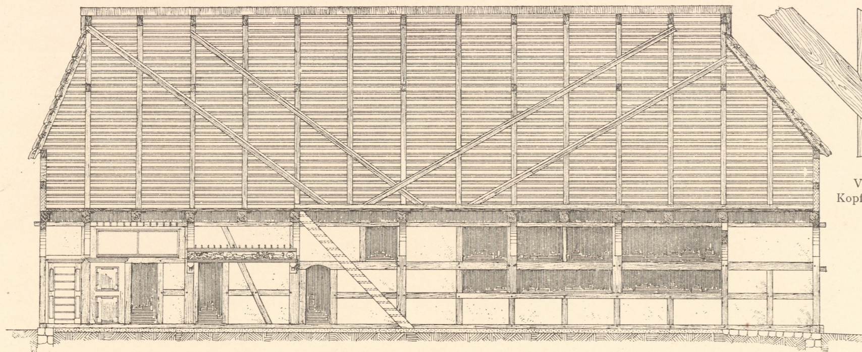
Abb. 2. Längenschnitt a-b.
