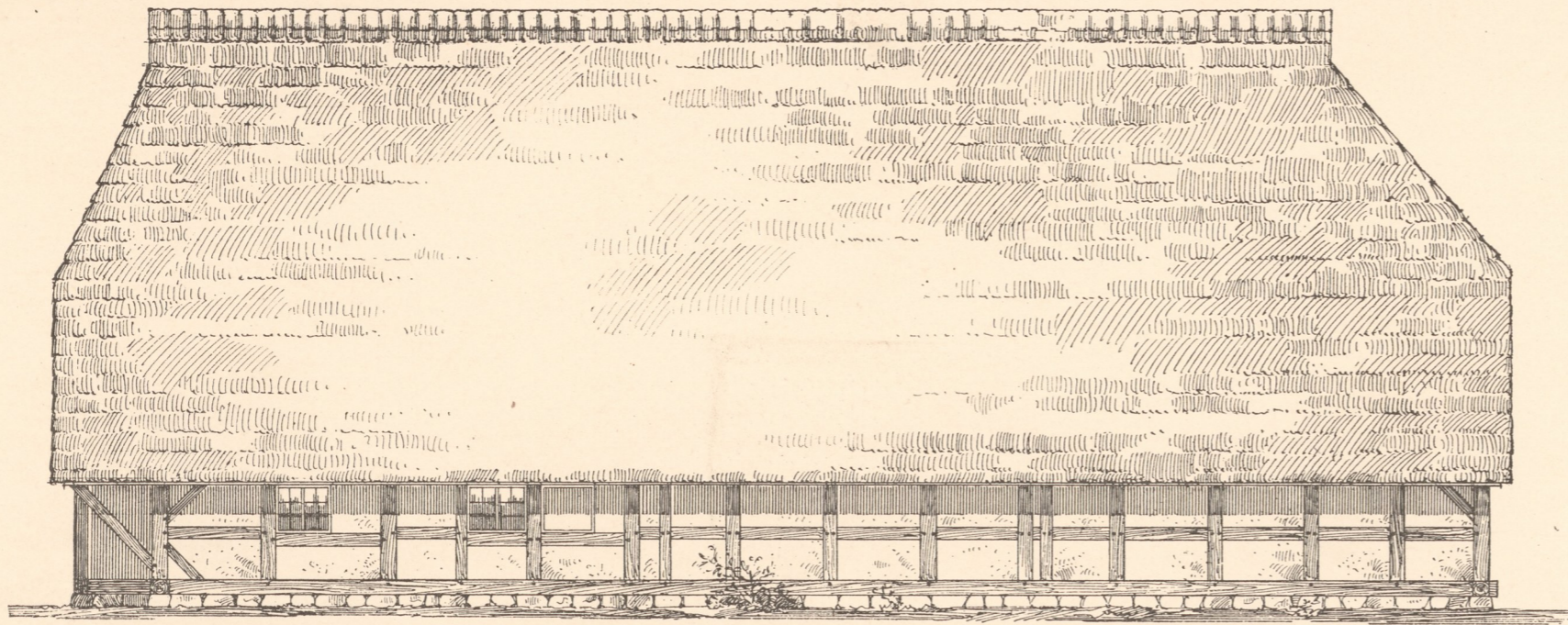
Abb. 1. Seitenansicht.
