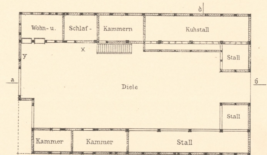
Abb. 5. Grundriss.
