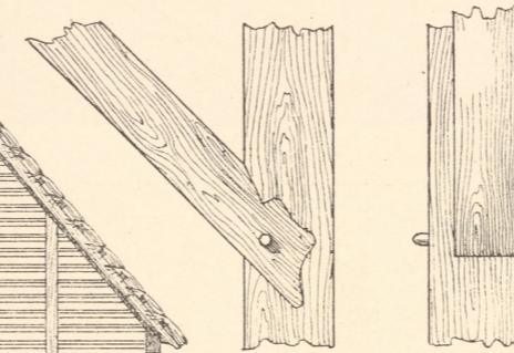
Abb. 7. Verbindung von Kopfband u. Ständer.
