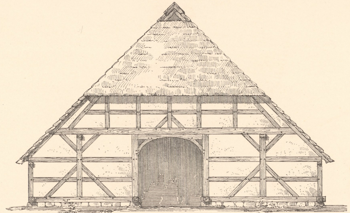
Abb. 3. Giebelansicht.
