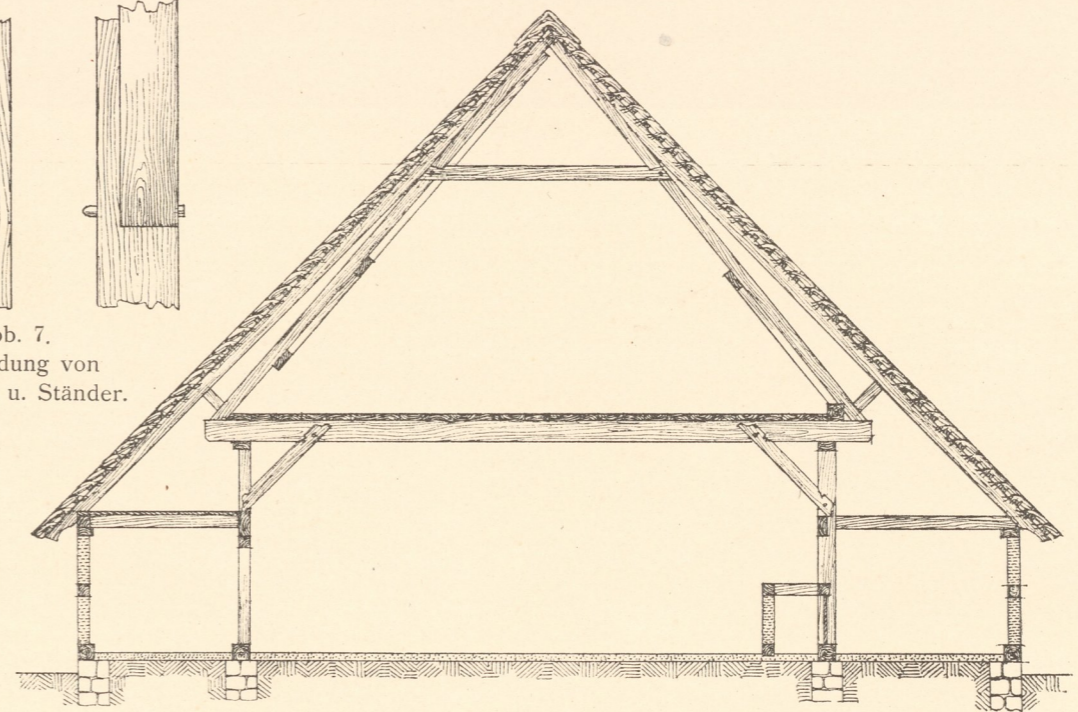
Abb. 4. Querschnitt c-d.
