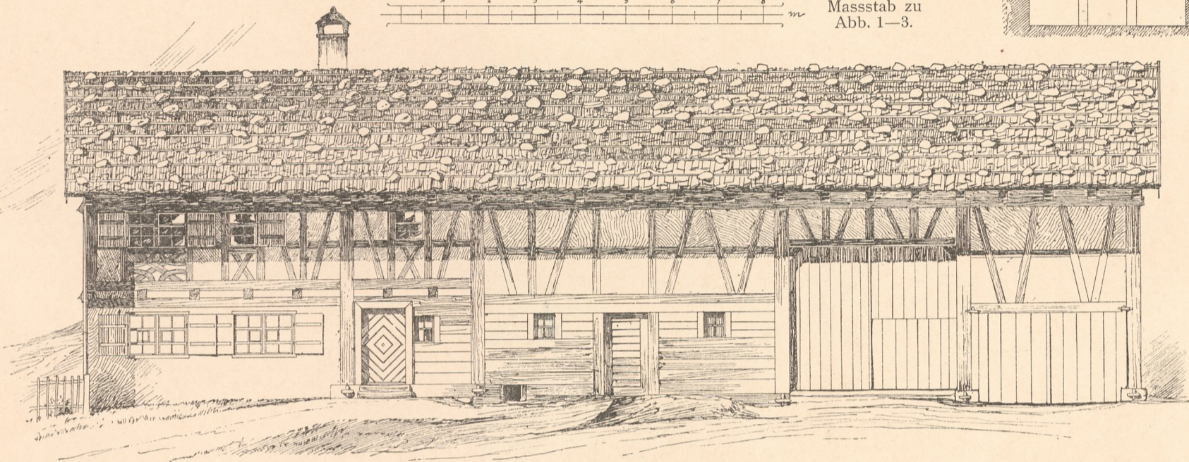
Abb. 3. Waffenried, Südseite.
