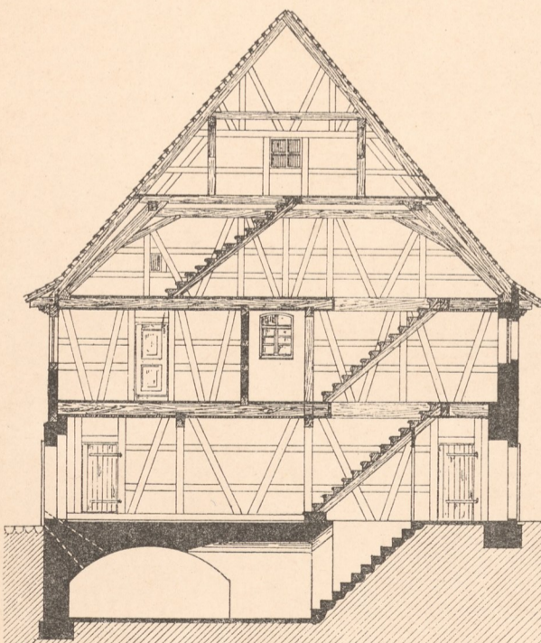
Abb. 8. Unter-Aspach, Schnitt.
