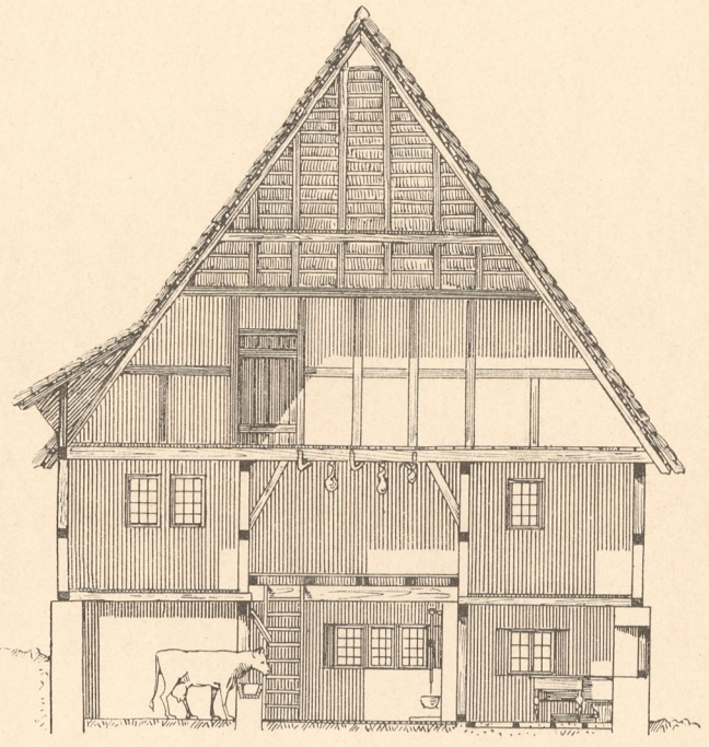
Abb. 3. Immecke, Querschnitt.
