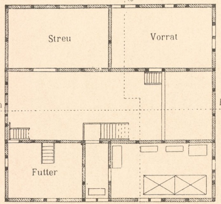
Abb. 5. Immecke, Stockwerk.
