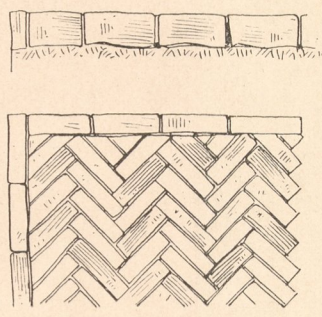
Abb. 17. Dielenpflaster.
