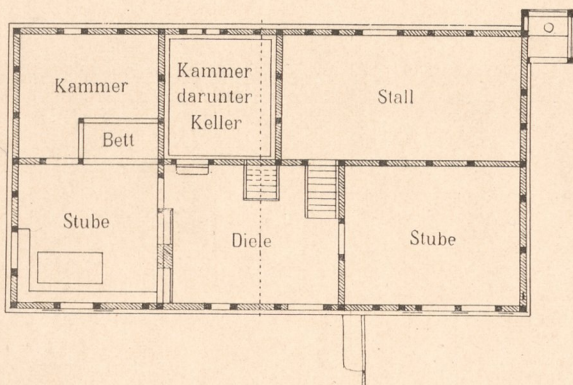
Abb. 15. Volmerhausen, Erdgeschoss.
