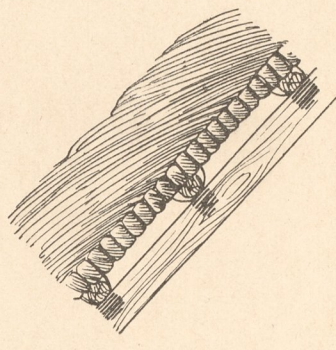
Abb. 18. Strohdeckung.
