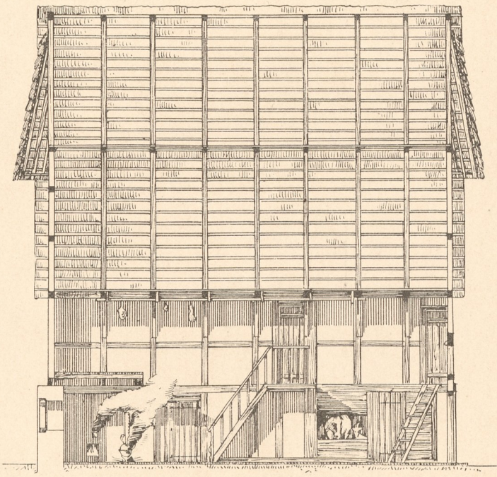
Abb. 4. Immecke, Längenschnitt.
