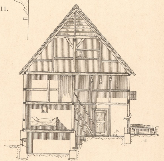
Abb. 14. Volmerhausen, Querschnitt.
