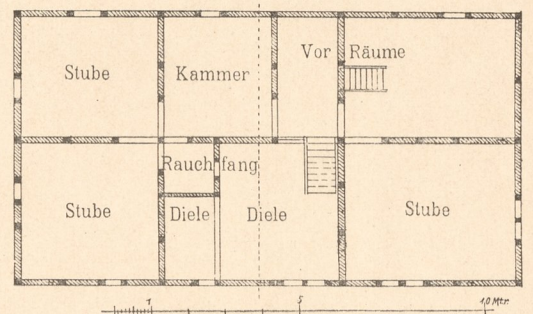
Abb. 16. Volmerhausen, Stockwerk.
