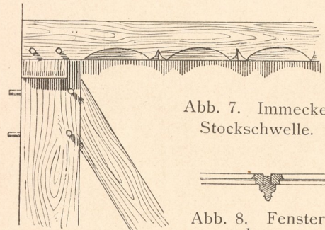
Abb. 7—11. Masstab 1 : 20.
