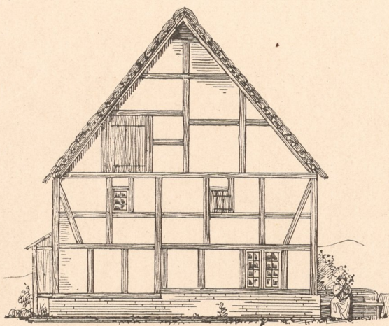
Abb. 12. Volmerhausen, Giebelansicht.
