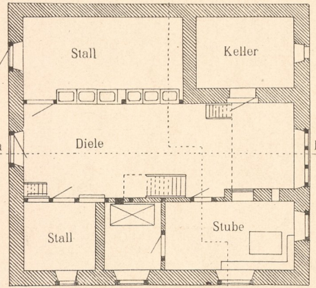
Abb. 6. Immecke, Erdgeschoss.
