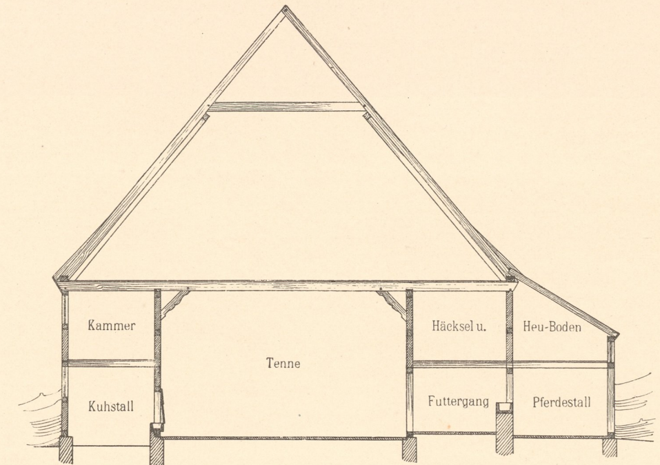
Abb. 4. Querschnitt.
