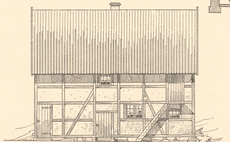
Abb. 6. Backhaus.
