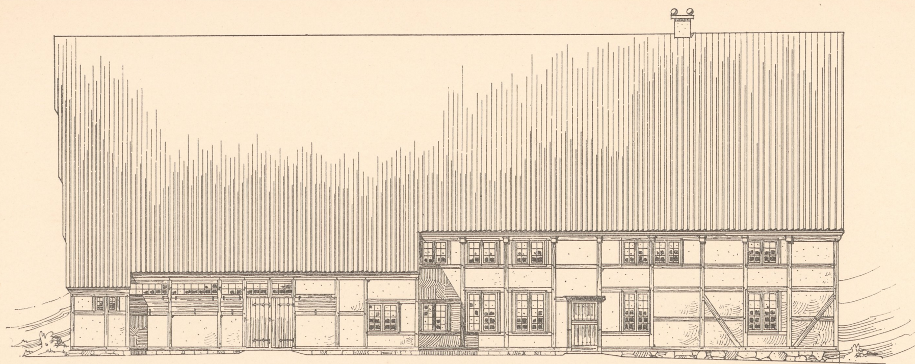
Abb. 1. Längsansicht.
