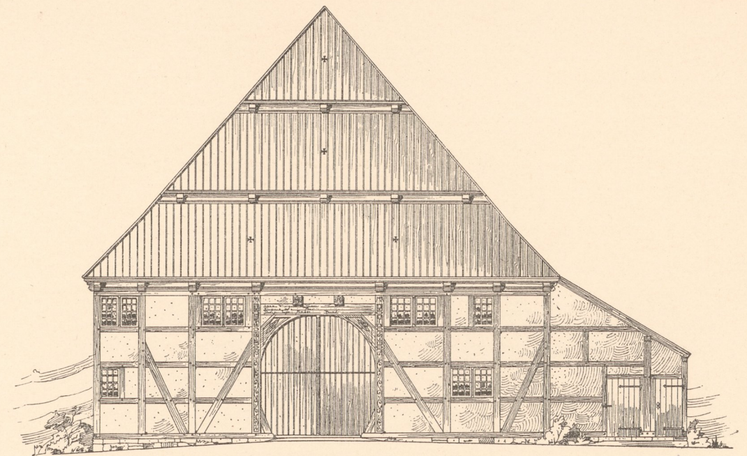
Abb. 2. Giebelansicht.
