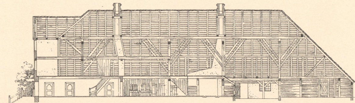
Abb. 13. Hochdorfer Hauberg. Längenschnitt.
