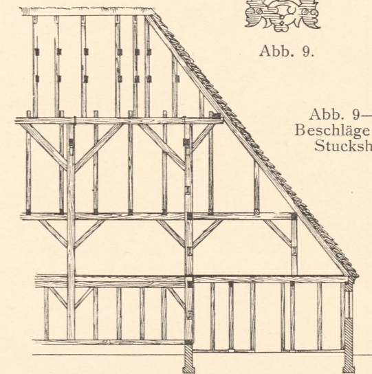
Abb. 6. Rother Hauberg. Längenschnitt.
