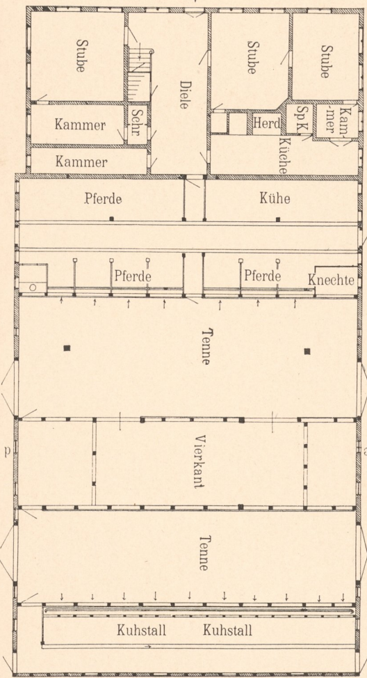
Abb. 12. Haus Dyrsen in Norderdeich.
