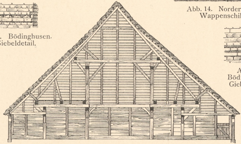
Abb. 13. Haus Dyrsen in Norderdeich. Querschnitt c d.
