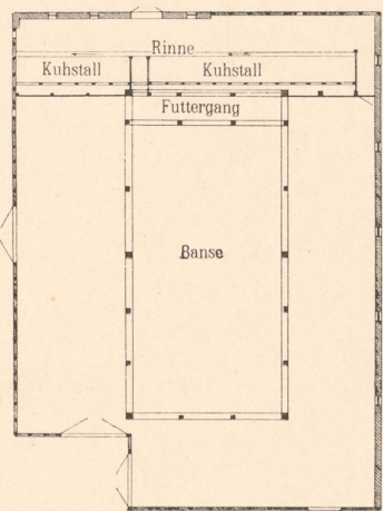
Abb. 17. Haubergscheune in Barlte Altendeich.
