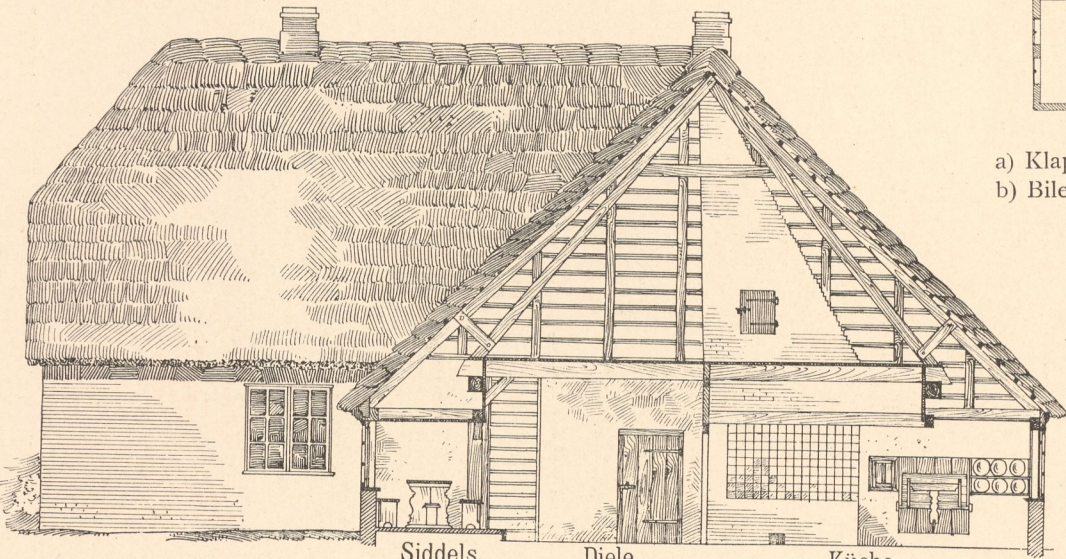
Abb. 2. Haus Groth in Bödinghusen. Querschnitt x y.
