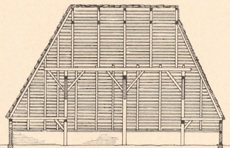
Abb. 10. Bödinghusen. Schnitt a b durch die Scheune.
