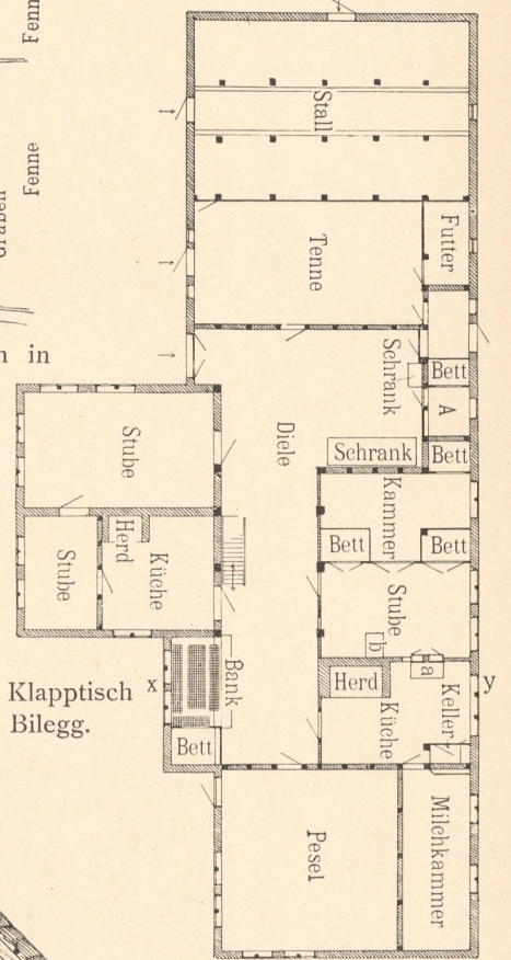
Abb. 4. Haus Groth in Bödinghusen. Grundriss.
