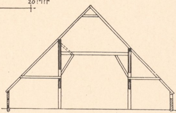
Abb. 16. Haubergscheune in Barlte Altendeich. Querschnitt.
