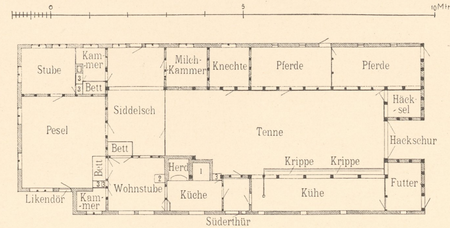
Abb. 13. Haus Thiessen in Schmedeswurth bei Marne.
