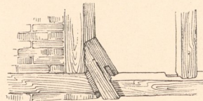
Lehe. Thürschwelle und Pfosten.
