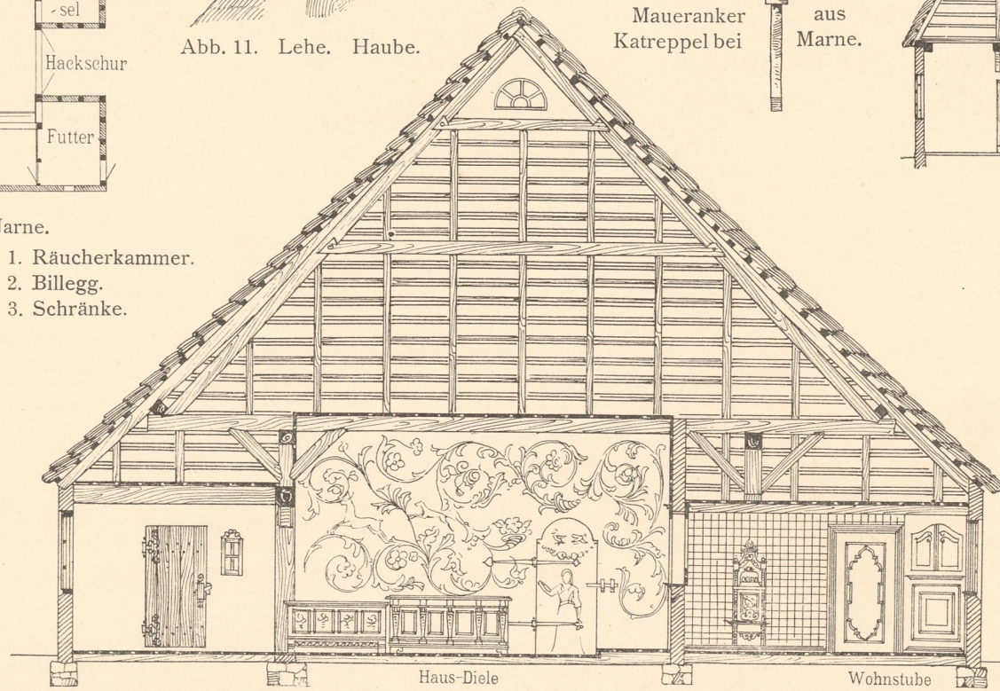
Abb. 15. Haus Thiessen in Schmedeswurth bei Marne. Querschnitt.
