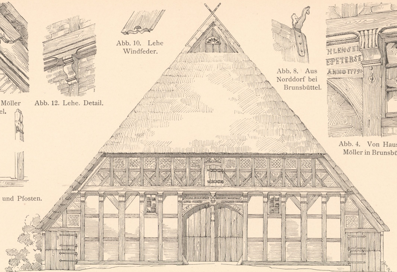
Abb. 6. Haus Claus Hinrichs in Lehe, 1775. Giebelansicht.
