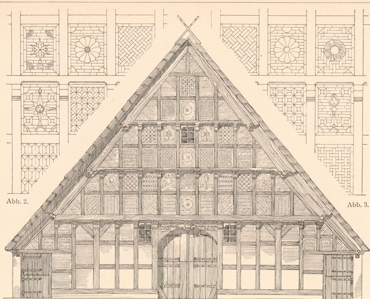
Abb. 1. Haus Möller in Brunsbüttel, 1779. Giebelansicht.
