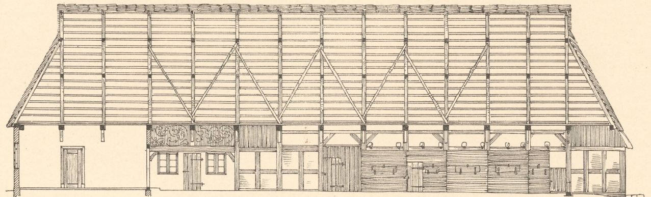
Abb. 14. Haus Thiessen in Schmedeswurth bei Marne. Längenschnitt.
