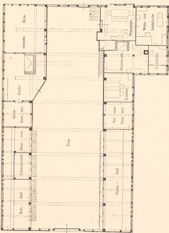
Abb. 4. Grundriss.
