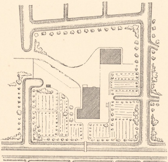
Abb. 5. Lageplan.
