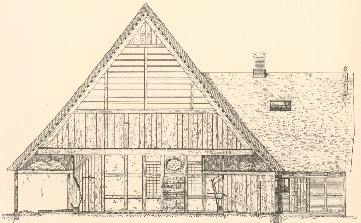
Abb. 3. Querschnitt durch Diele und Ställe.
