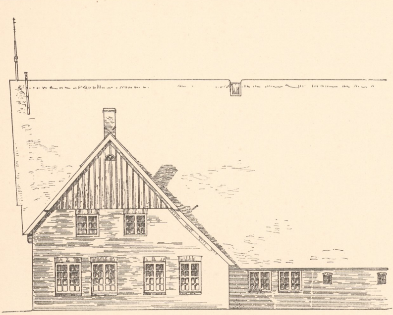
Abb. 1. Längensicht.
