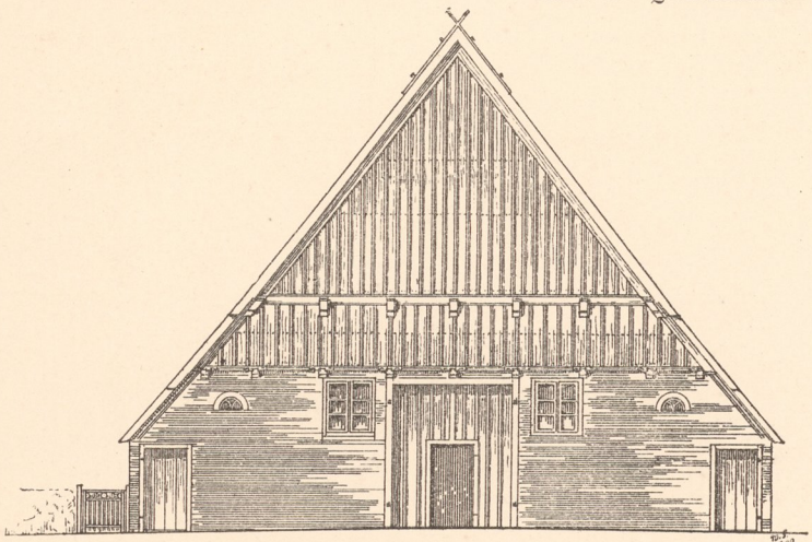
Abb. 5. Giebelansicht.
