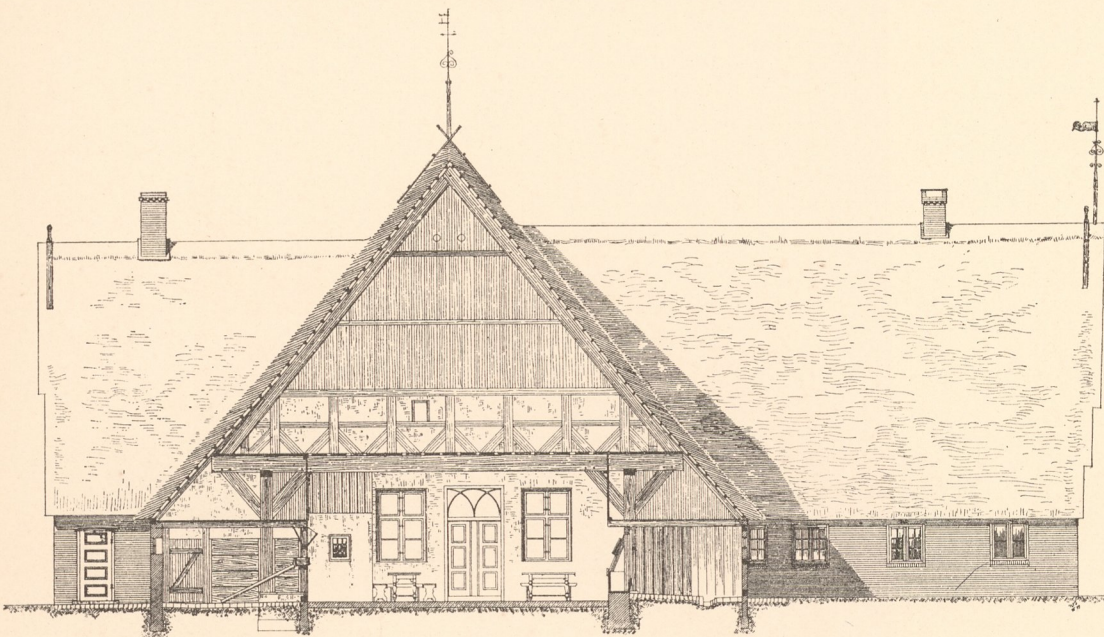
Abb. 3. Querschnitt.
