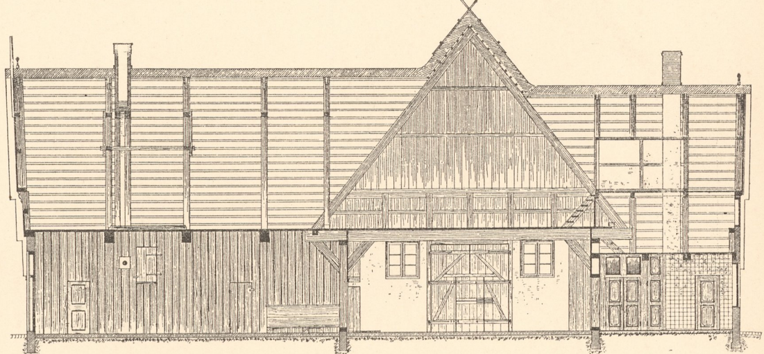
Abb. 6. Längenschnitt.
