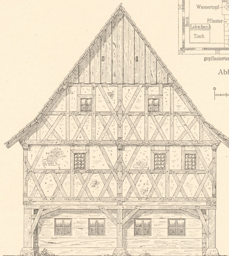
Abb. 7. Schenkendorf. Giebelansicht.
