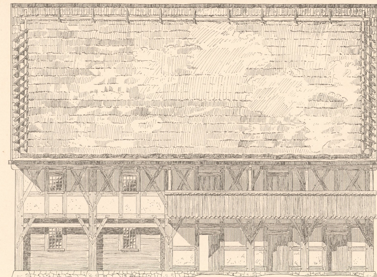
Abb. 2. Goldberg. Längsansicht.
