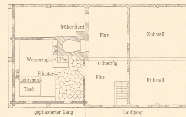
Abb. 4. Goldberg. Grundriss.
