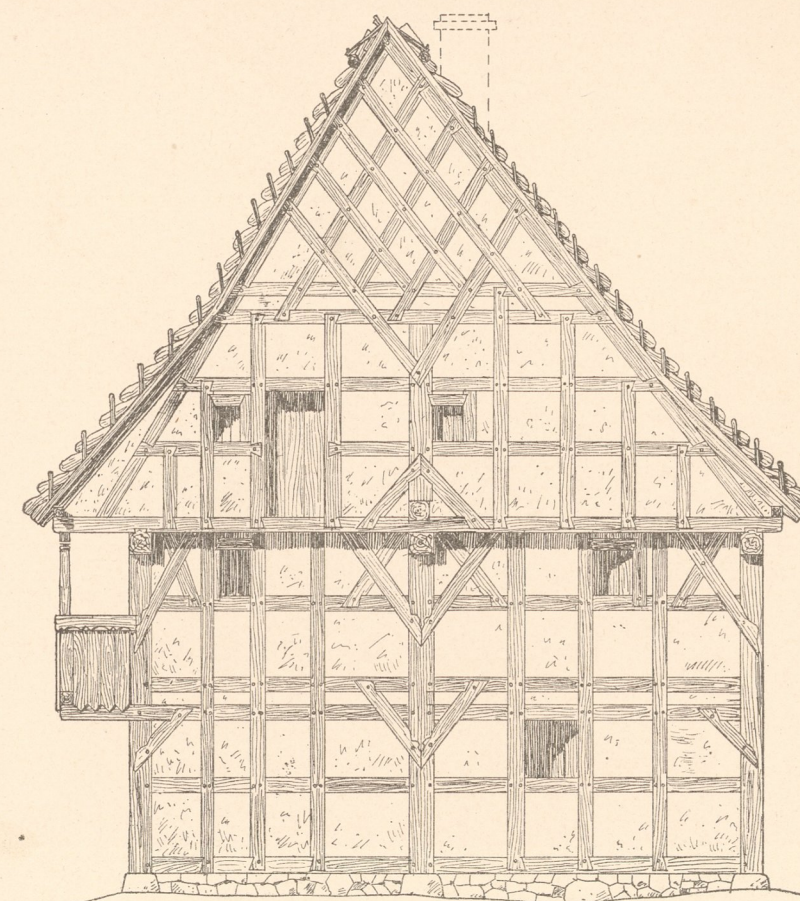
Abb. 3. Goldberg. Giebelansicht.
