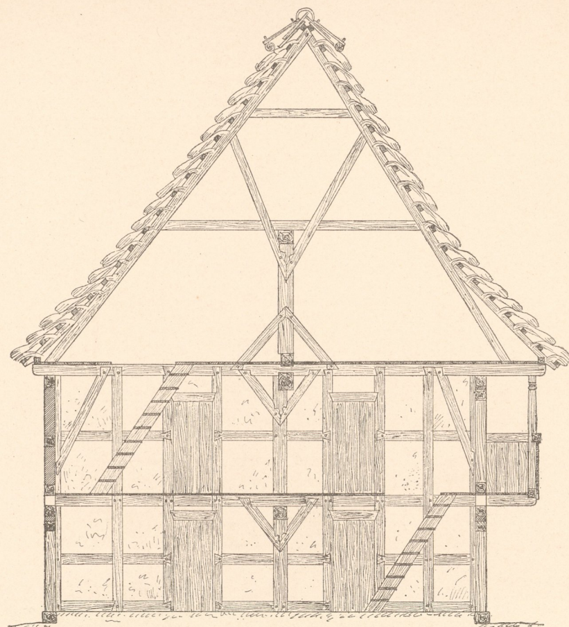
Abb. 1. Goldberg. Querschnitt.
