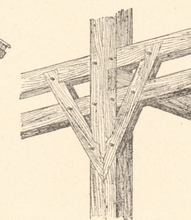
Abb. 5. Goldberg. Einzelheit.
