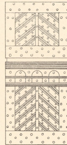
Abb. 9. Thür aus Unter-Schöna. 1:30.
