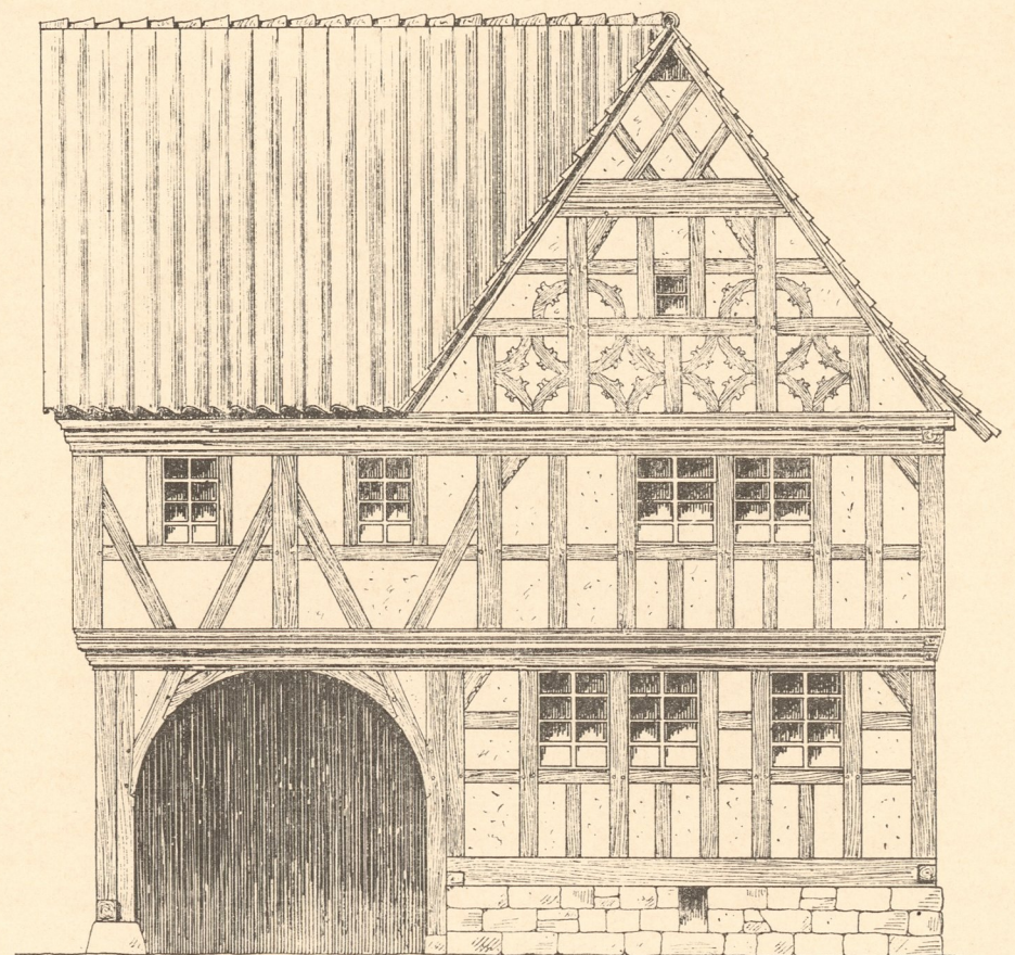
Abb. 5. Bauernhaus No. 37 in Simmershausen (S.-Meiningen, Kr. Hildburghausen).
