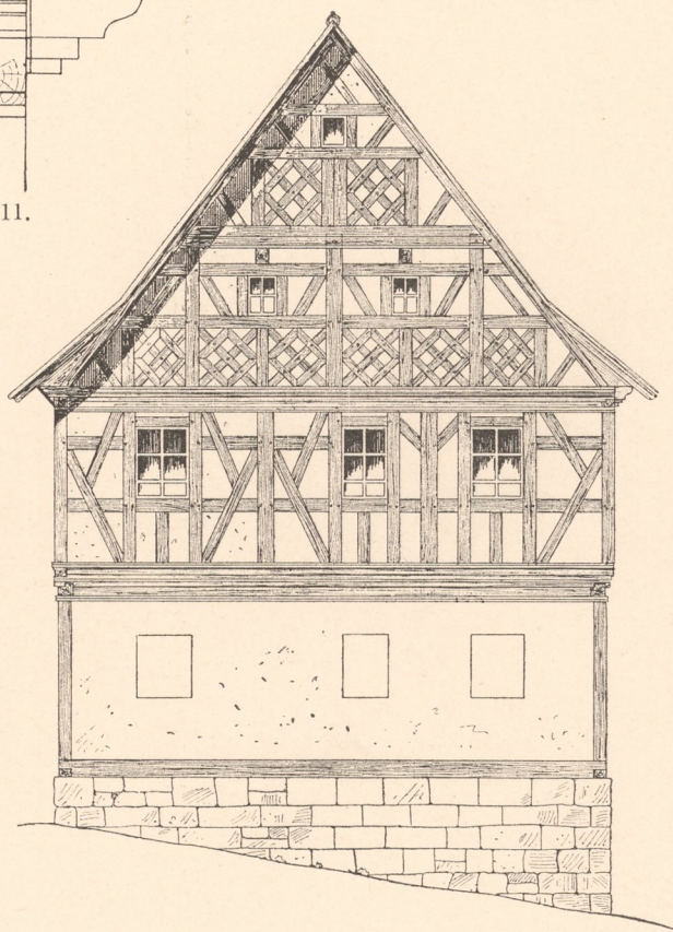
Abb. 4. Bauernhaus No. 35 aus Mönchröden, Giebelseite.
