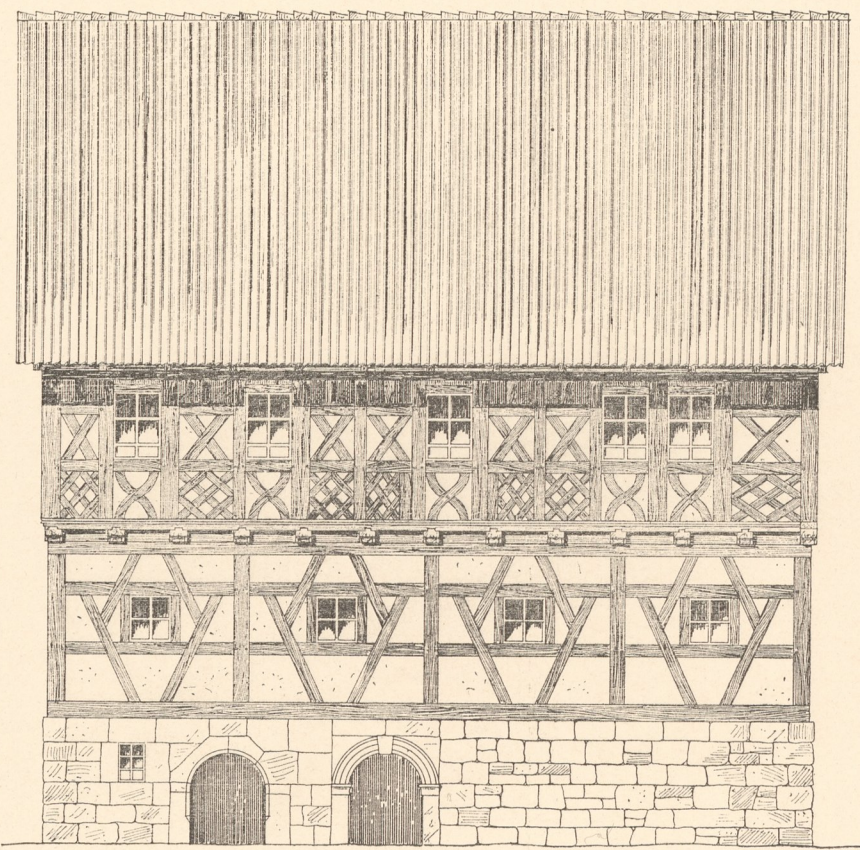
Abb. 5. Bauernhaus No. 35 aus Mönchröden, Langseite.
