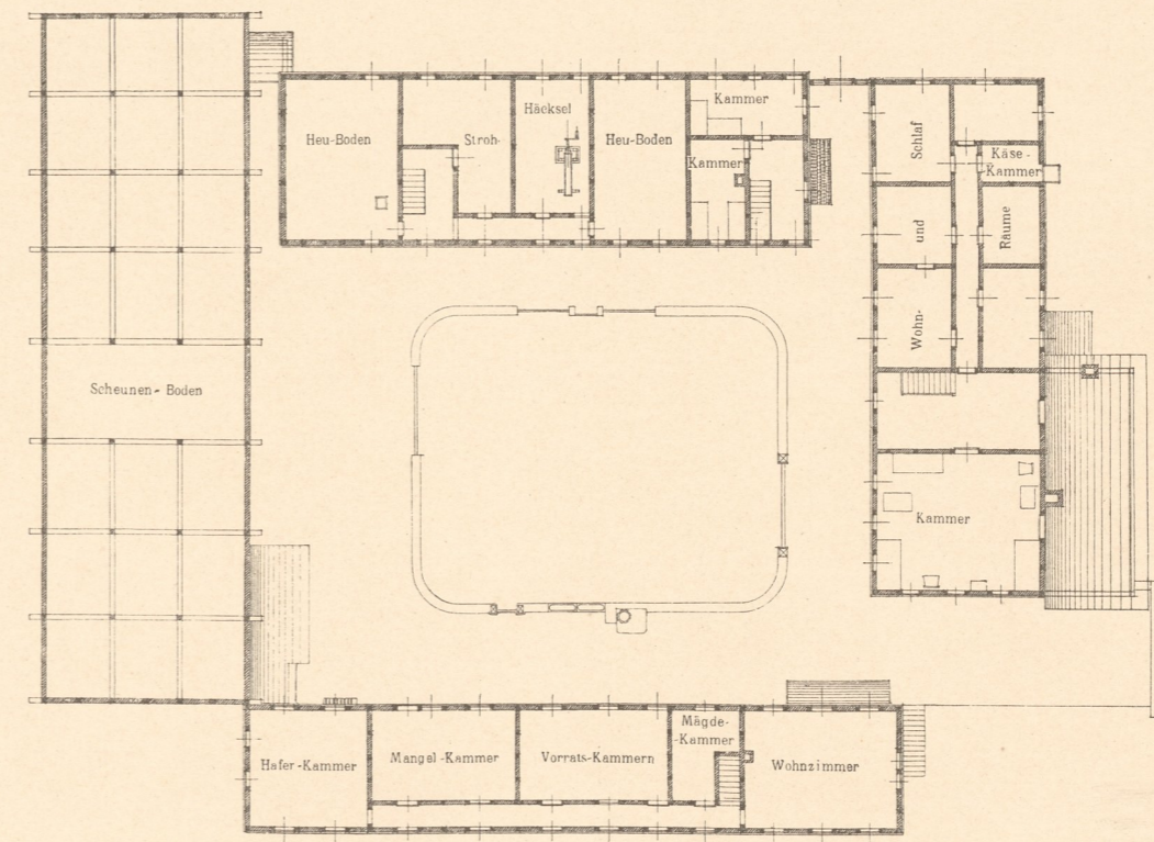
Abb. 4. Grundriss vom Obergeschoss.
