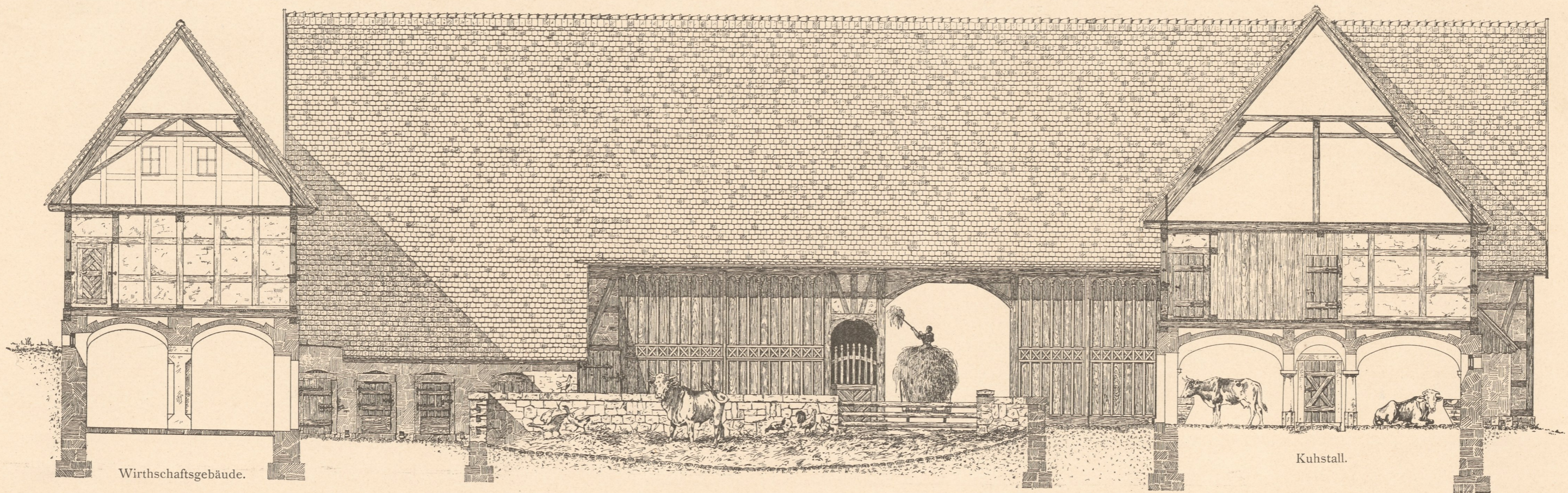
Ansicht der Scheune.
