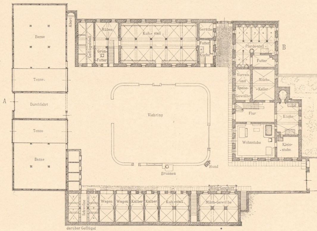
Abb. 3. Grundriss vom Erdgeschoss.
