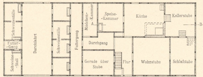
Abb. 10. Sallenthin. Grundriss des Wohnhauses.
