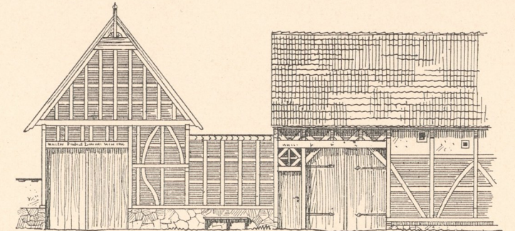
Abb. 17. Strassenseite des Pferdestalles.
