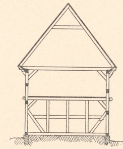
Abb. 17-19. Bauernhaus der Aug. Schulze Wwe. in Vissum.
