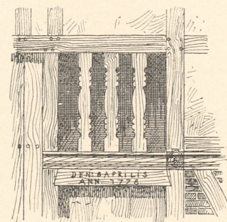
Abb. 14. Sallenthin. Detail des Einganges.
