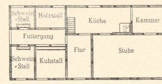
Abb. 11. Sallenthin. Grundriss des Altenteils.
