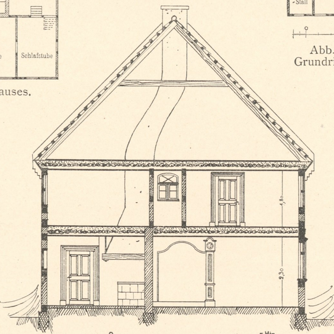
Abb. 2. R. Schulz in Vissum. Querschnitt a b durch das Wohnhaus.
