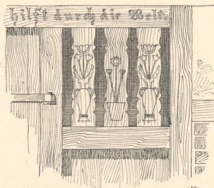
Abb. 15. Detail des Einganges. Abb. 15 und 16. Vom Kuhstall des Joachim Baade in Vissum, erb. 1825.
