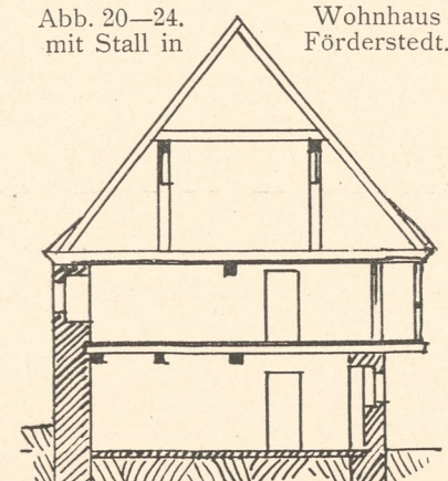
Abb. 23. Förderstedt. Schnitt e f.
