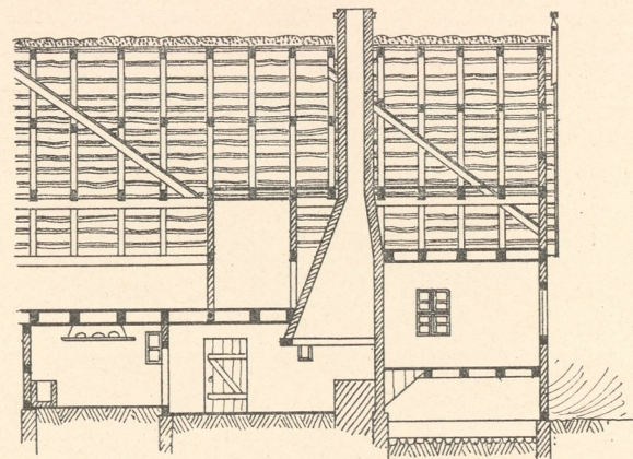
Abb. 8. Sallenthin. Schnitt A B.
