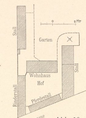
Abb. 19. A. Schulze Ww. in Vissum. Lageplan.
