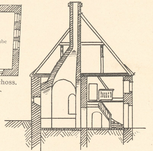
Abb. 22. Förderstedt. Schnitt a b.
