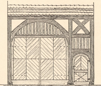
Abb. 12. Einfahrtsthor mit Pfortchen.
