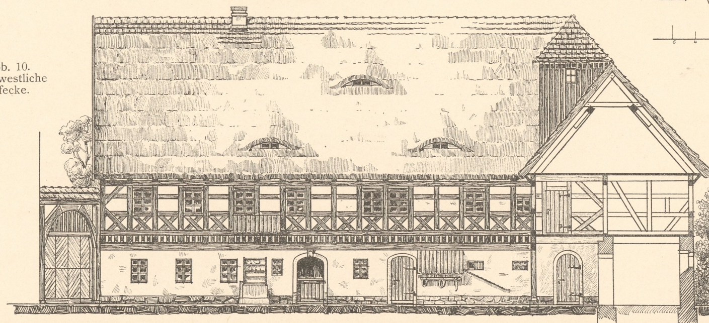
Abb. 11. Wohnhaus. Ostfront.
