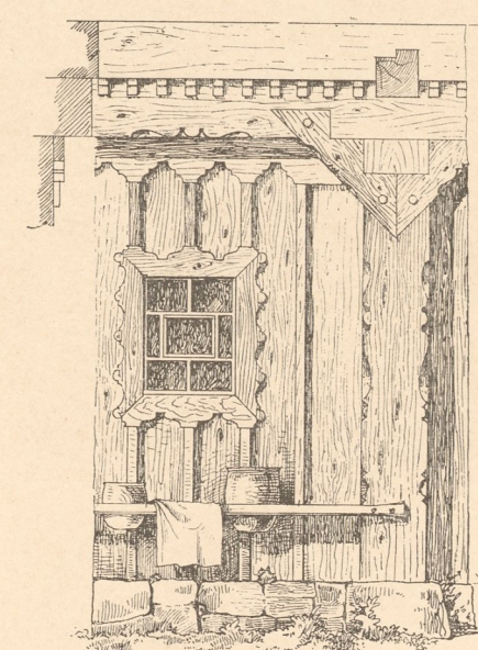
Abb. 13. Hölzerne Umfassungswand.
