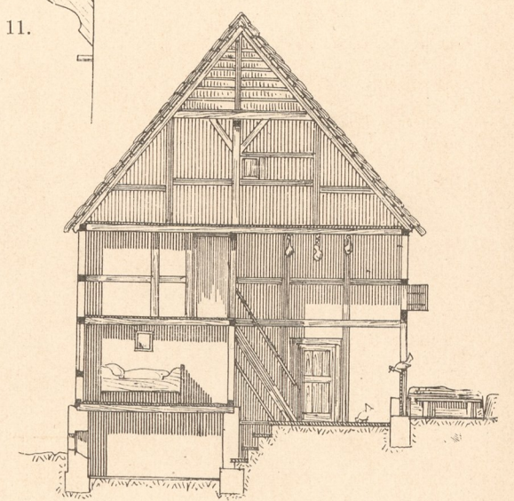
Abb. 14. Volmerhausen, Querschnitt.
