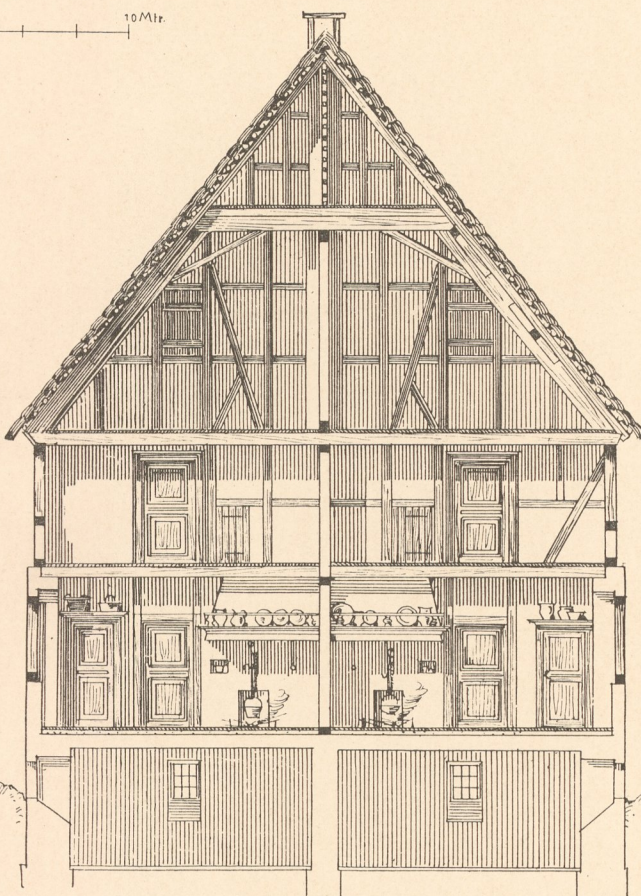
Abb. 3. Liefenroth, Querschnitt.
