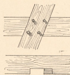
Abb. 15. Lohmar, Bohlenstrebe.
