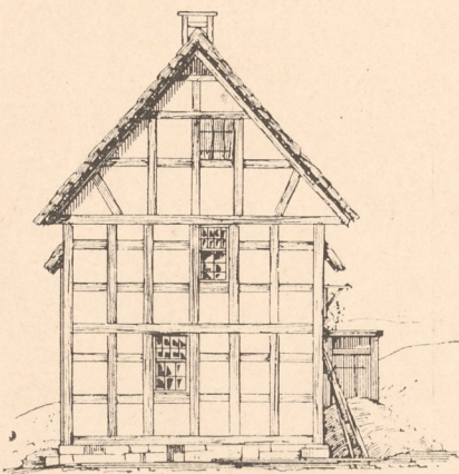
Abb. 10. Lohmar, Giebelansicht.
