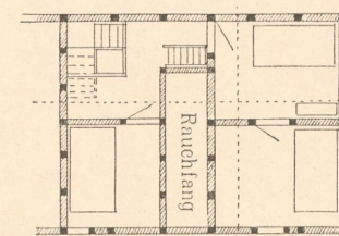
Abb. 14. Lohmar, Oberstock.
