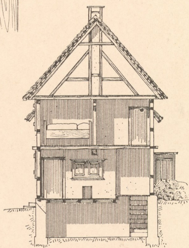
Abb. 11. Lohmar, Querschnitt.
