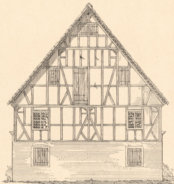
Abb. 2. Liefenroth, Giebelansicht.
