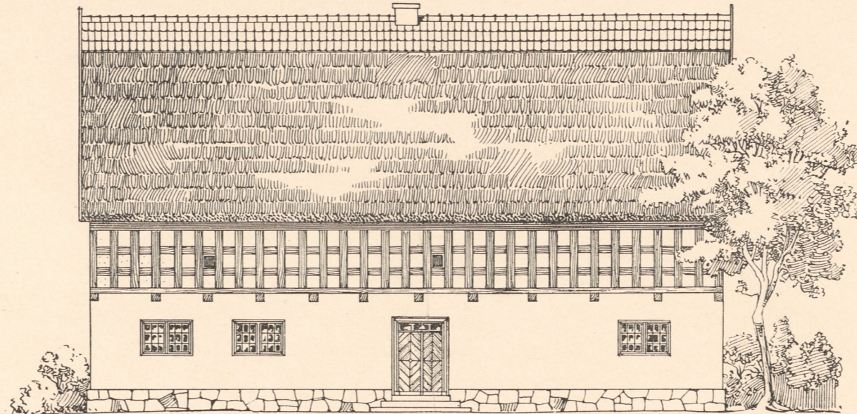
Abb. 1. Ermländisches Wohnhaus für einen Grossbauern. Strassenseite.
