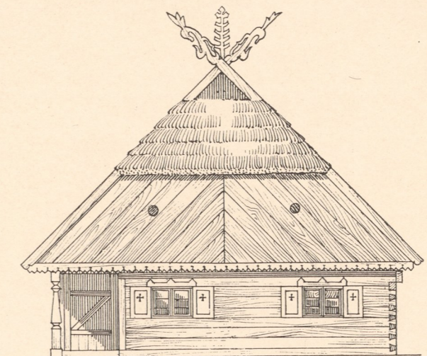
Abb. 8. Giebelansicht.
