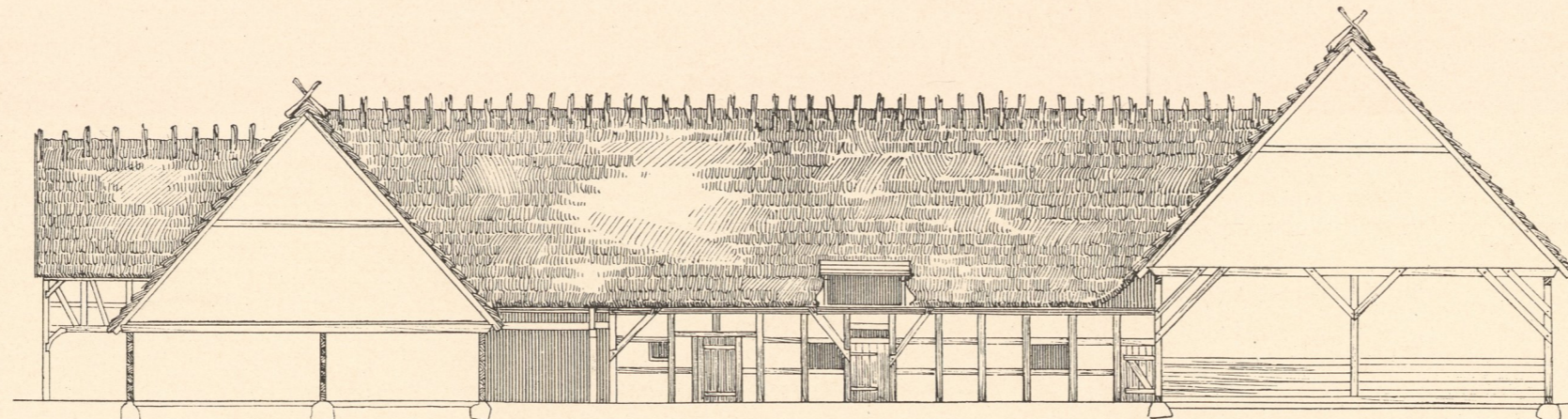
Abb. 4. Gehöft eines Grossbauern in Ebersbach bei Braunsberg. Längenschnitt durch das Gehöft.
