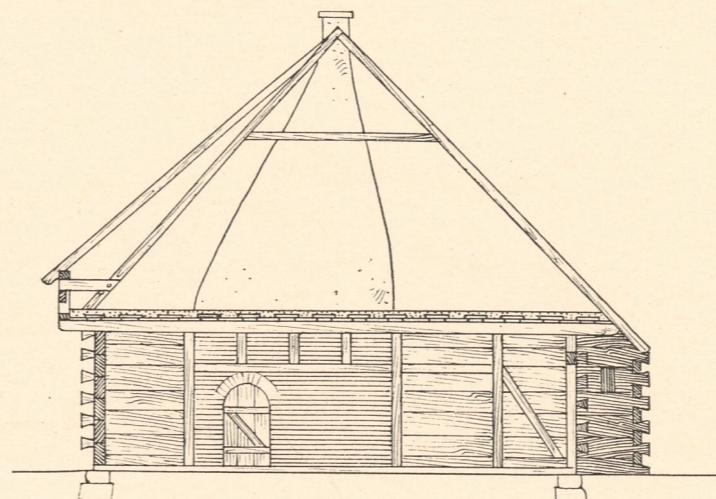
Abb. 7. Querschnitt a b.
