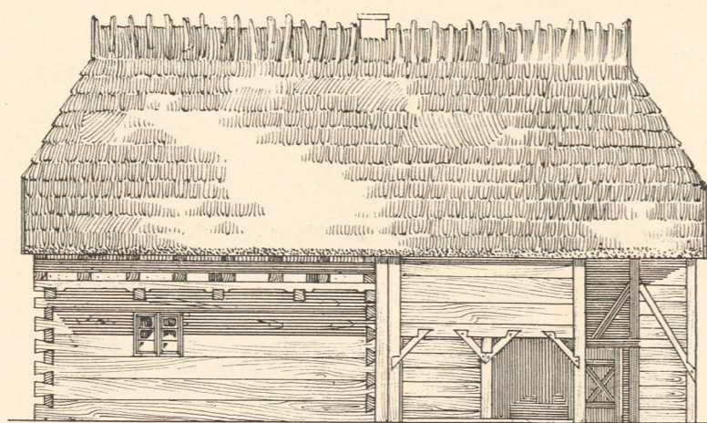
Abb. 6. Längsansicht. Strassenseite.
