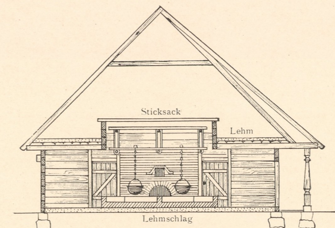
Abb. 9. Querschnitt.
