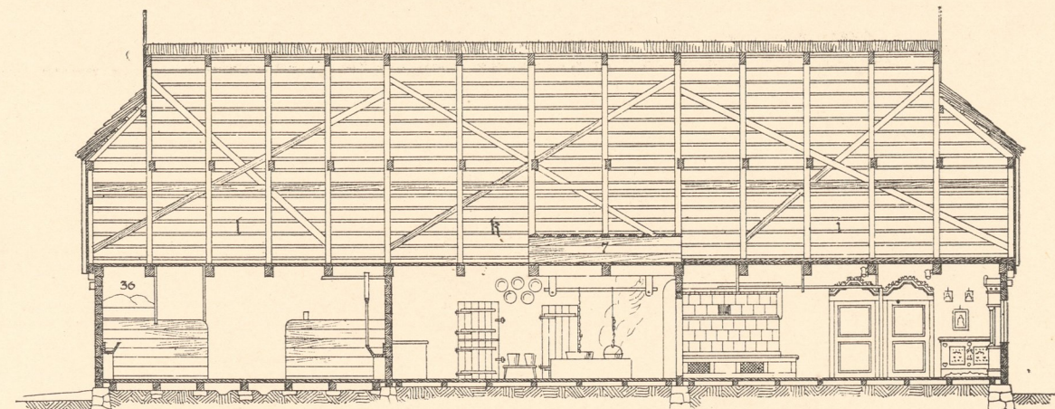
Abb. 3. Wohnhaus, Längenschnitt.
