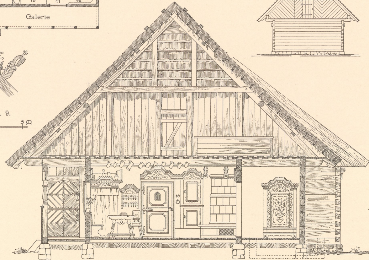
Abb. 5. Wohnhaus, Querschnitt.
