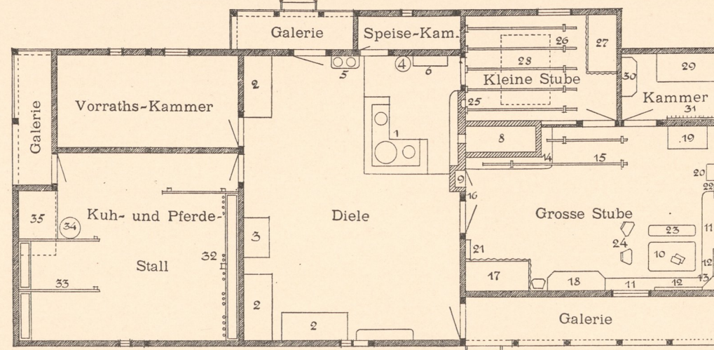
Abb. 1. Wohnhaus, Erdgeschoss.
