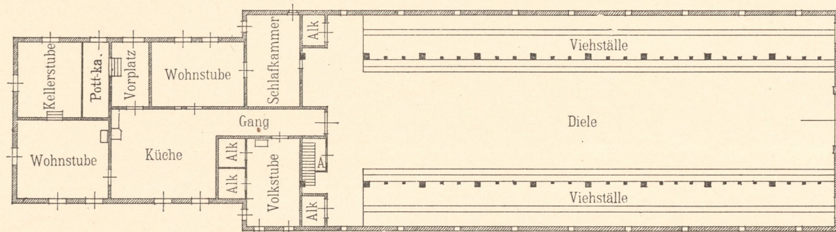
Abb. 5. Osterseefeld. Grundriss.
