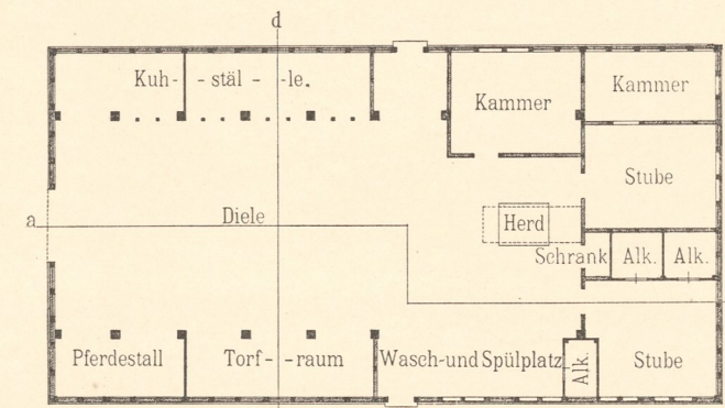
Abb. 6. Mansholt. Grundriss.
