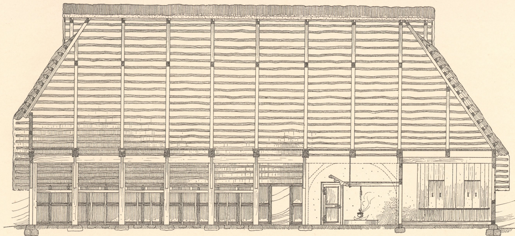
Abb. 3. Mansholt. Längenschnitt a b.
