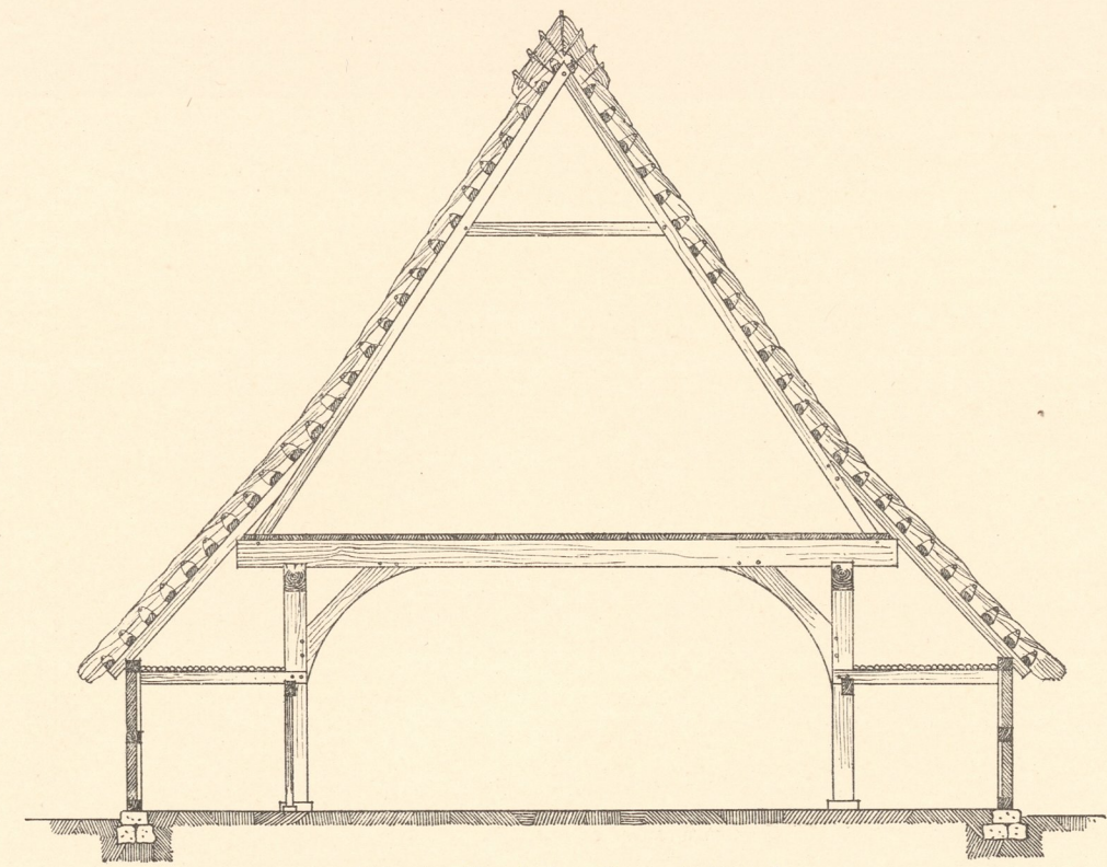
Abb. 4. Mansholt. Querschnitt c d.
