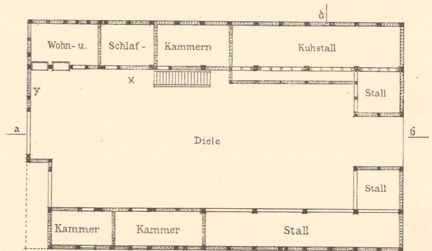
Abb. 5. Grundriss.
