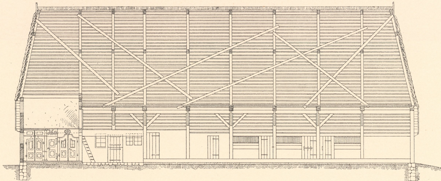
Abb. 3. Längen-Schnitt a b.
