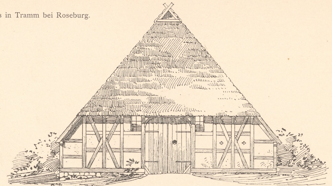
Abb. 2. Vorder-Ansicht.
