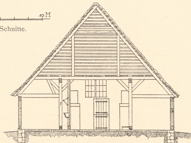
Abb. 7. Querschnitt c d.
