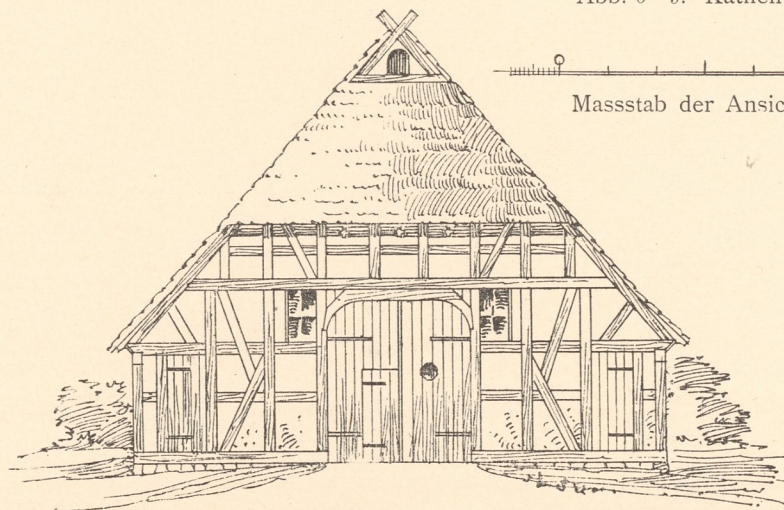
Abb. 6. Vorder-Ansicht.
