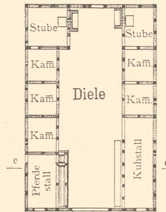
Abb. 8. Grundriss.
