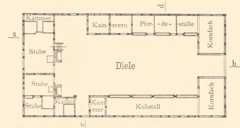
Abb. 5. Grundriss.
