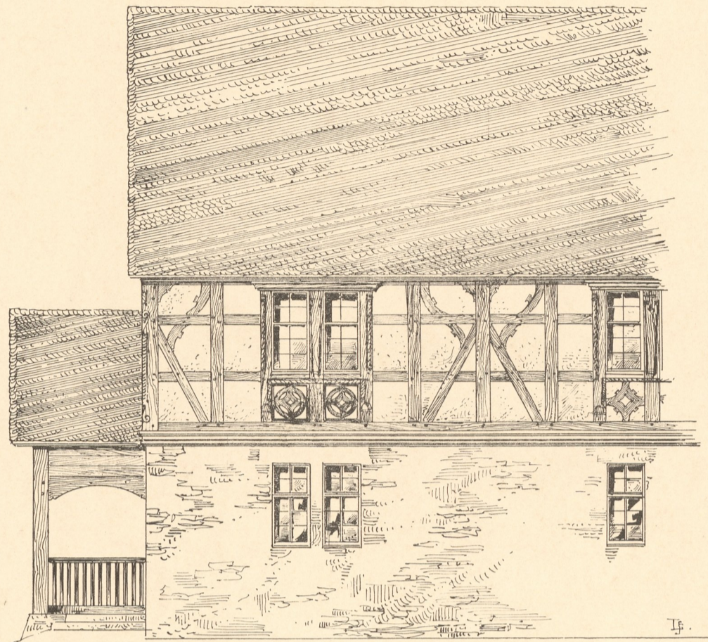
Abb. 2. Langseite.
