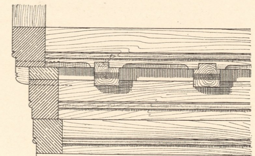
Abb. 6. Détail von der Hofseite der Thoreinfahrt.
