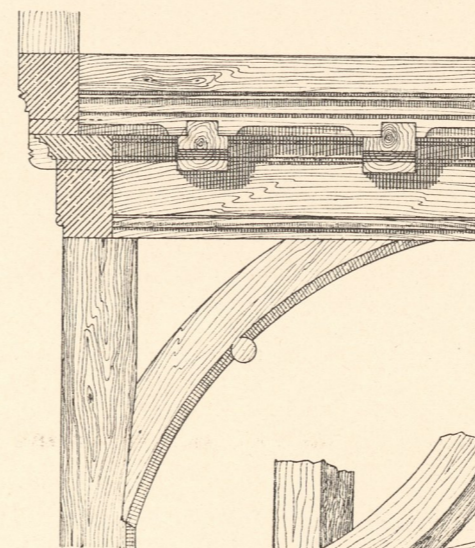
Abb. 2. Haus des P. Maurer in Brandobendorf. Ansicht der Strassenseite vom Wohn- und Thorhaus.
