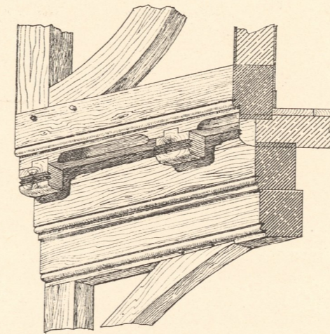
Abb. 7. Gebälk der Strassenseite. Jüngerer Theil.
