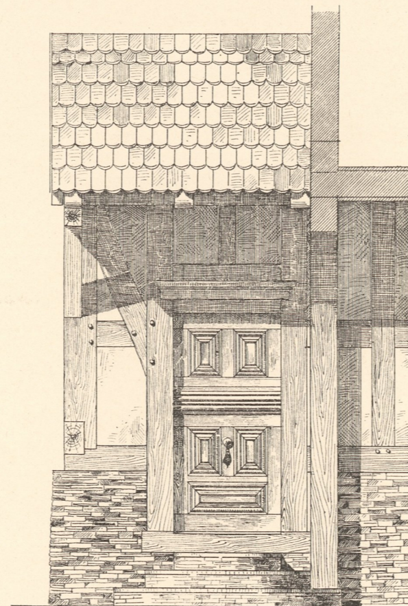
Abb. 4. Haus Maurer in Brandobendorf. Détail der Hausthür.
