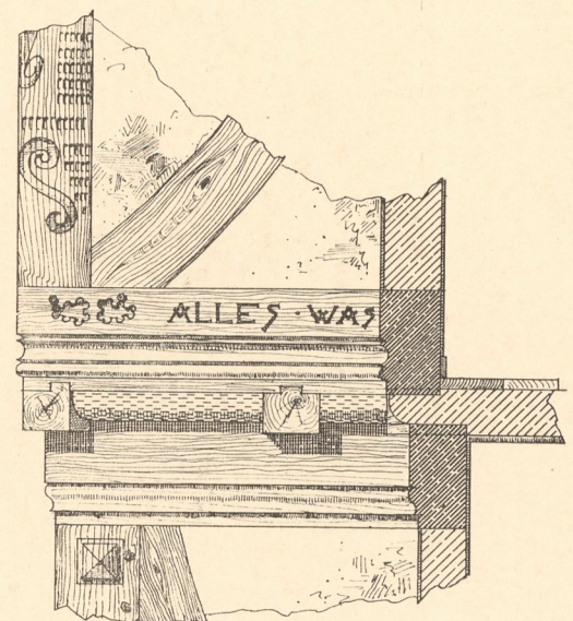
Abb. 8. Haus Maurer in Brandobberndorf. Gebälk an der Strassenseite. Aelterer Theil.
