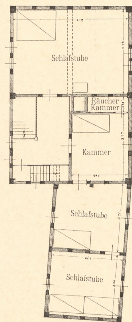
Haus Maurer in Brandobberndorf. Wohn- und Thorhaus. Grundriss vom I. Stock.
