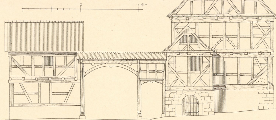
Abb. 6. Bauerngehöft Nr. 37 in Fronhausen (Kr. Marburg).
