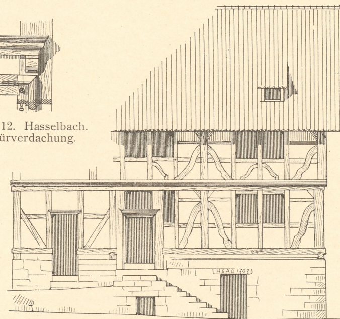
Abb. 11. Haus Nr. 18 in Hasselbach (Kr. Witzenhausen). Langseite.
