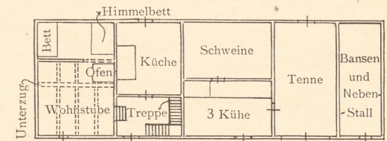
Abb. 5. Körle Nr. 36. Grundriss.
