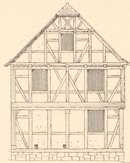
Abb. 1. Bauernhaus Nr. 5 in Körle (Kr. Melsungen). Giebelseite.
