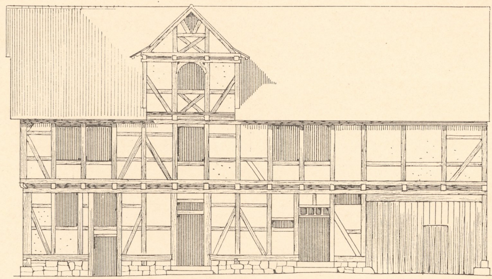
Abb. 2. Bauernhaus Nr. 5 in Körle (Kr. Melsungen). Langseite.
