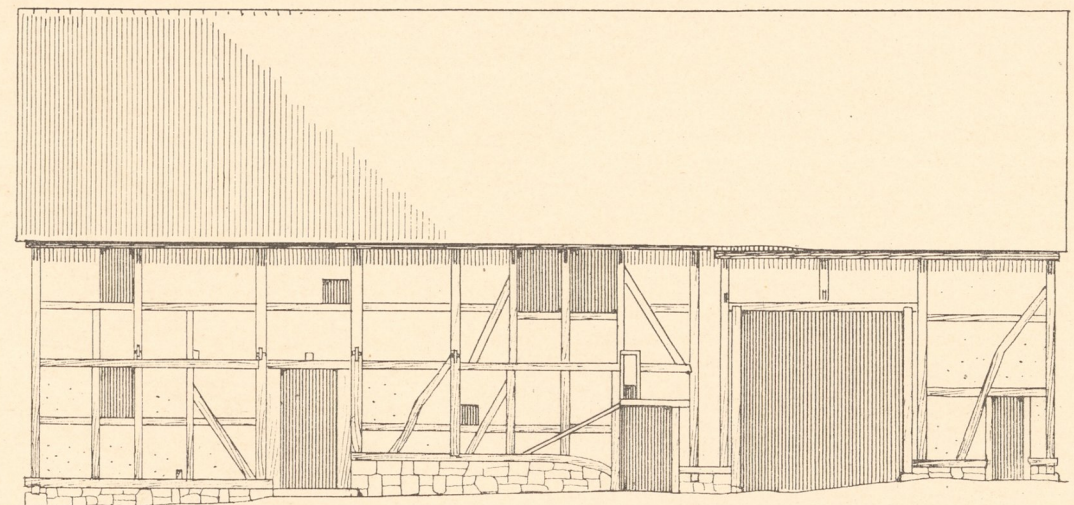
Abb. 3. Bauernhaus Nr. 36 in Körle (Kr. Melsungen). Langseite.
