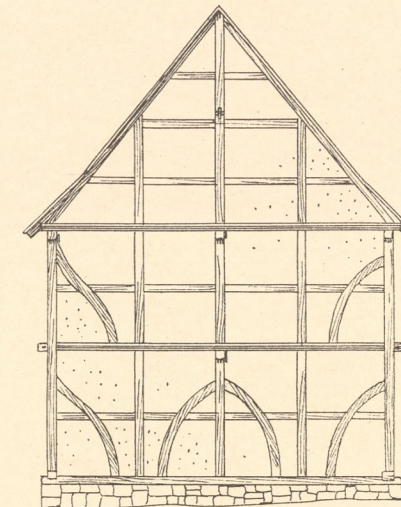
Abb. 4. Bauernhaus Nr. 36 in Körle (Kr. Melsungen). Giebelseite.
