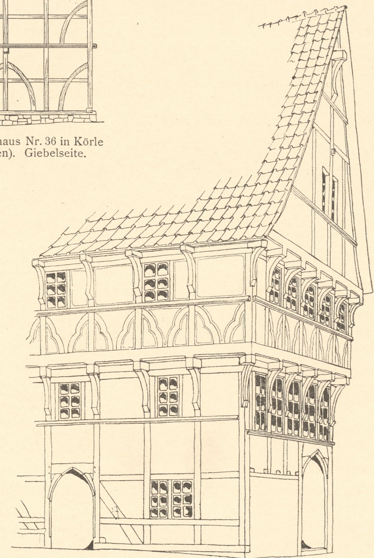
Abb. 13. Haus in der Entengasse in Witzenhausen.
