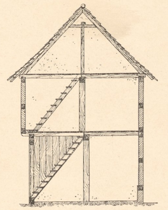
Abb. 6. Schnitt.
