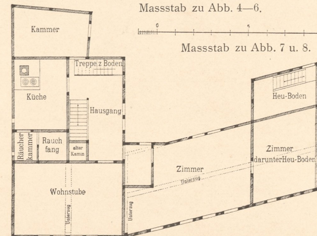
Abb. 7. Obergeschoss des Wohnhauses.
