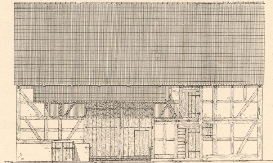
Abb. 4. Ansicht der Scheune.
