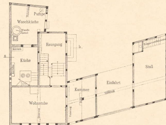
Abb. 8. Untergeschoss des Wohnhauses.
