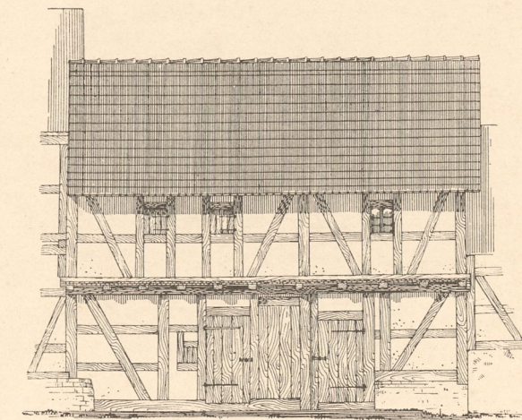
Abb. 5. Ansicht.
