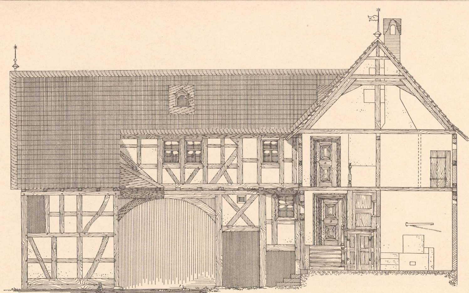
Abb. 1. Ansicht nach dem Hofe und Schnitt ba.
