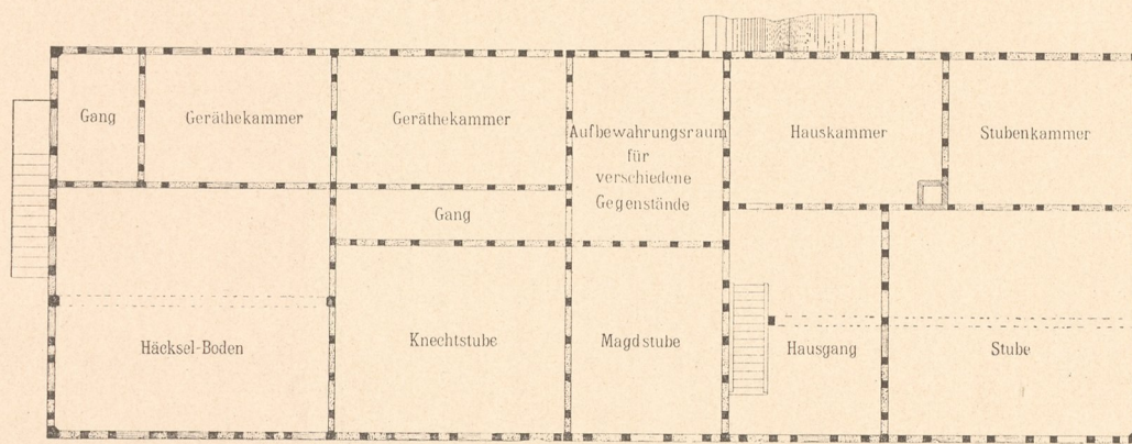
Abb. 4. Grundriss vom oberen Stock.
