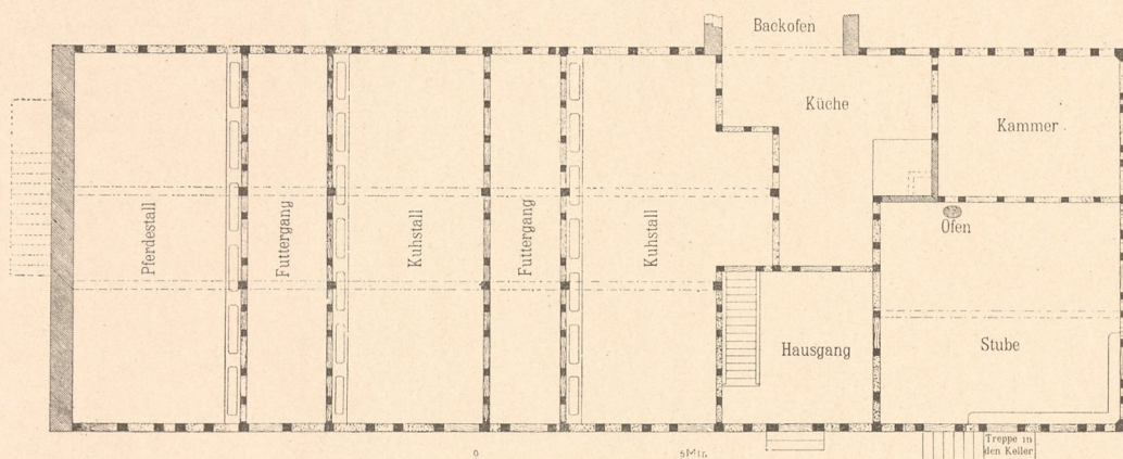
Abb. 5. Grundriss vom unteren Stock.
