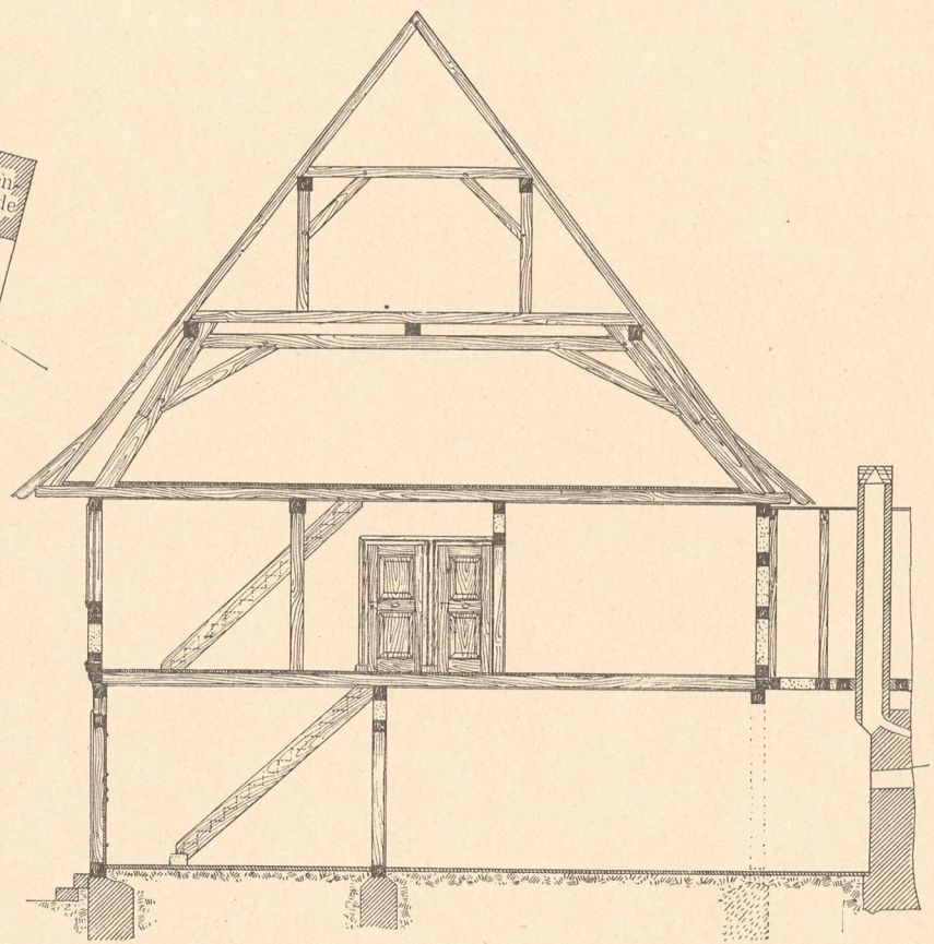
Abb. 3. Querschnitt.
