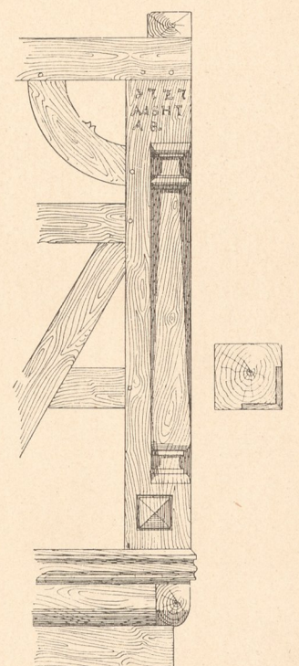
Abb. 8. Eckpfosten.
