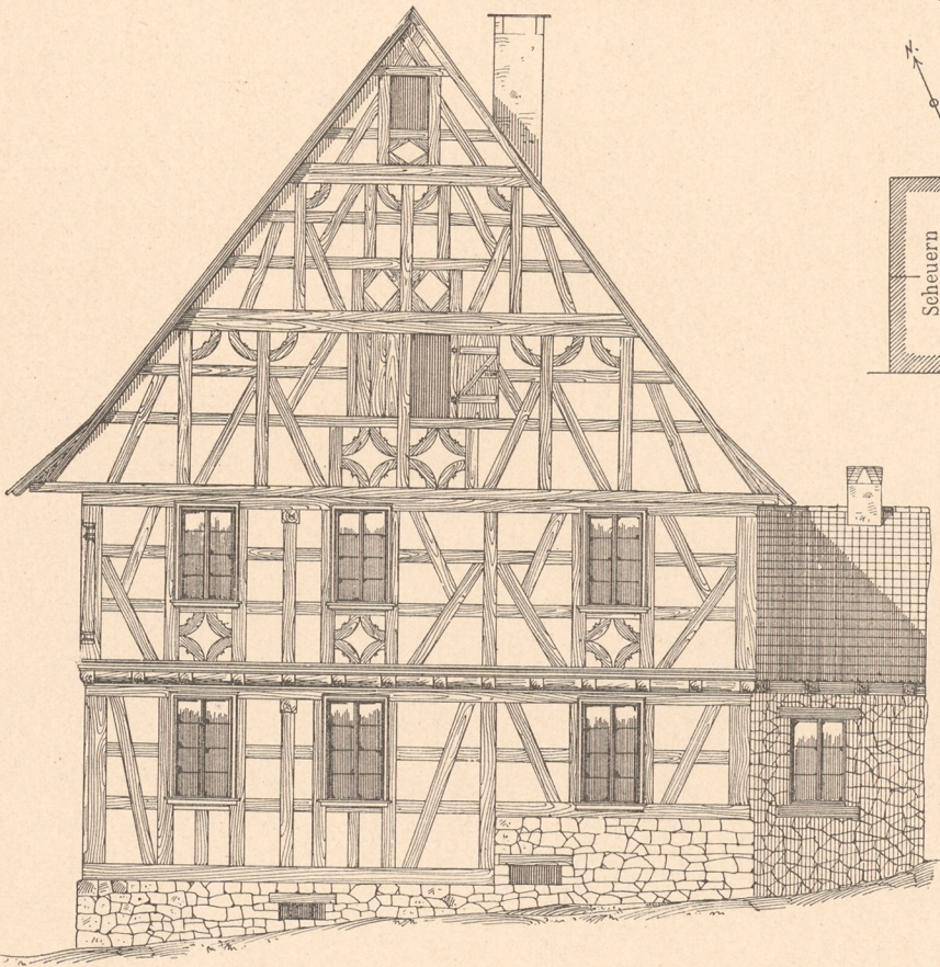
Abb. 2. Giebelansicht.
