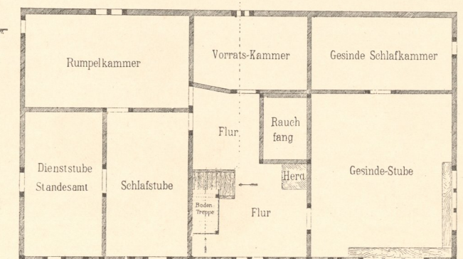
Abb. 11. Obergeschoss.
