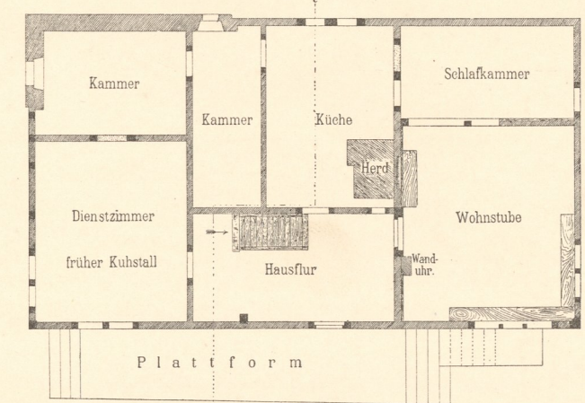
Abb. 12. Erdgeschoss.
