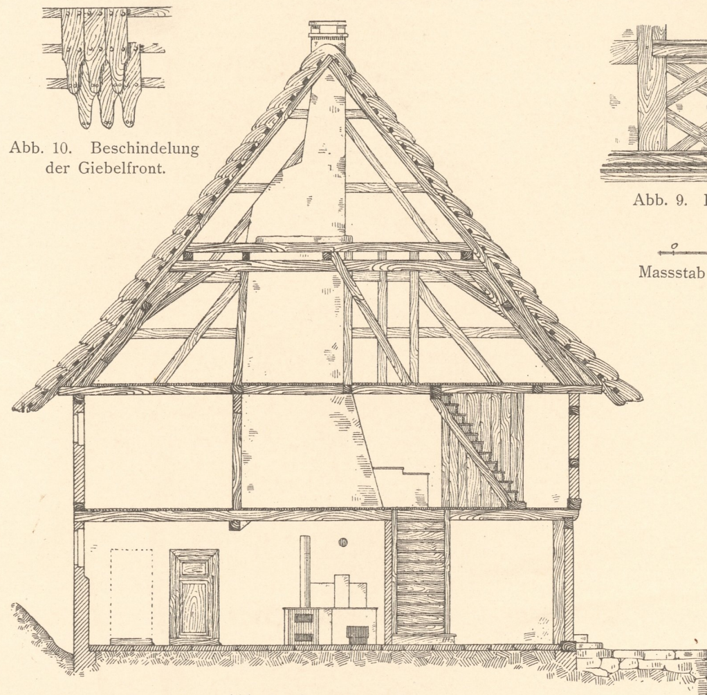
Abb. 2. Querschnitt CD.
