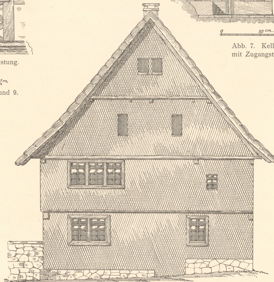
Abb. 3. Giebelansicht.
