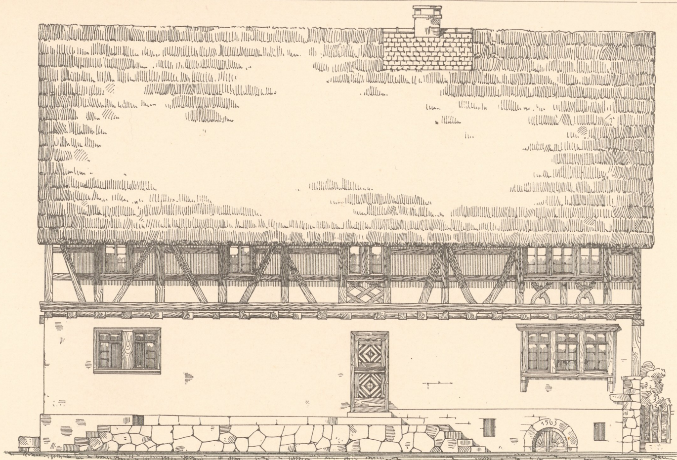
Abb. 1. Längsansicht.
