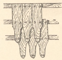
Abb. 10. Beschindelung der Giebelfront.
