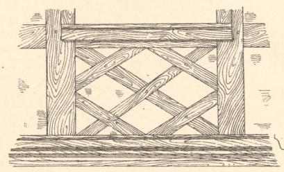
Abb. 9. Fachwerkbrüstung.
