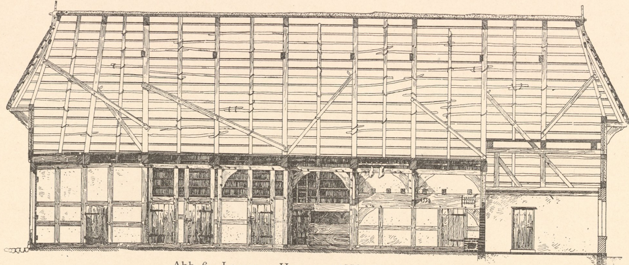
Abb. 6. Loccum. Haus von 1558. Längenschnitt.
