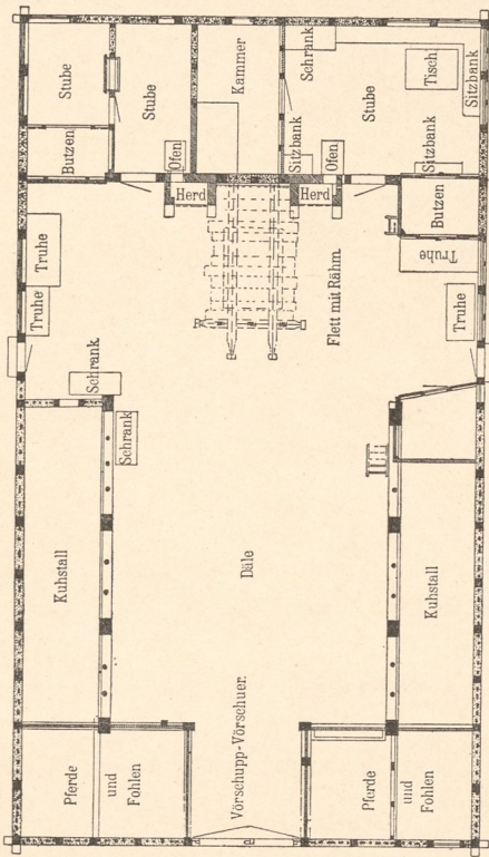
Abb. 11. Brackel. Grundriss.
