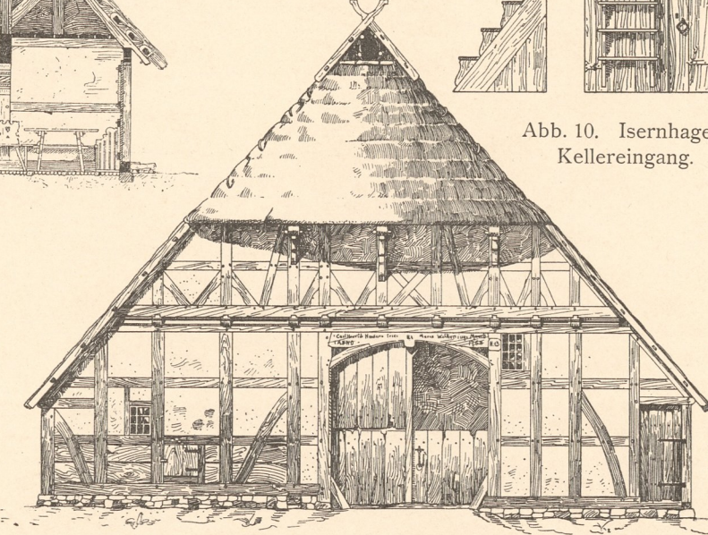
Abb. 14. Loccum. Haus von 1558. Giebelseite.
