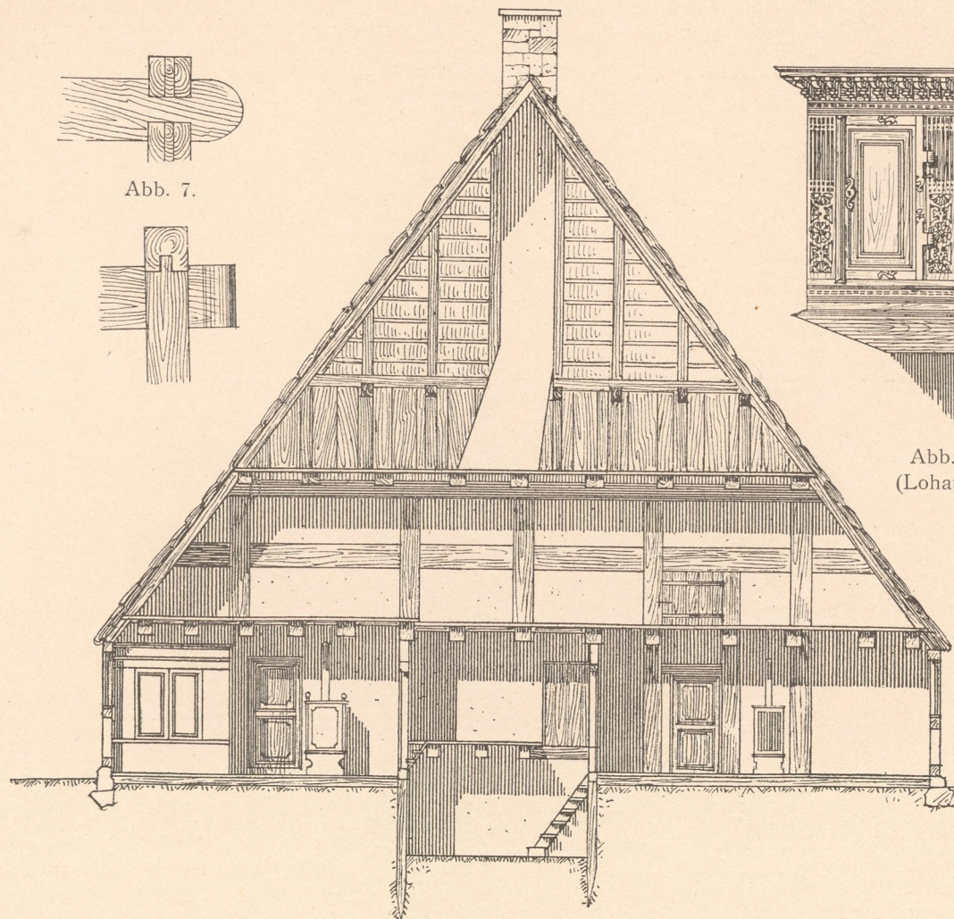
Abb. 1. Querschnitt c d.
