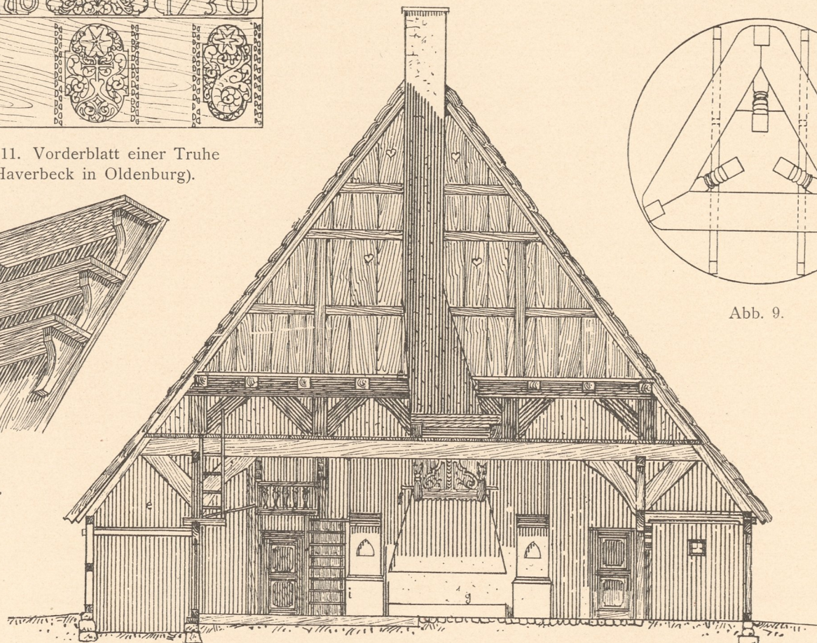
Abb. 3. Querschnitt a b.
