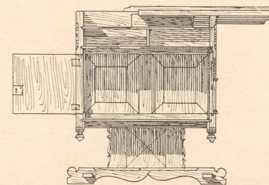
Abb. 9. Querschnitt.
