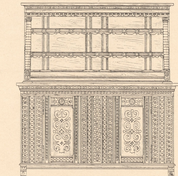
Abb. 4. Vorderansicht.
