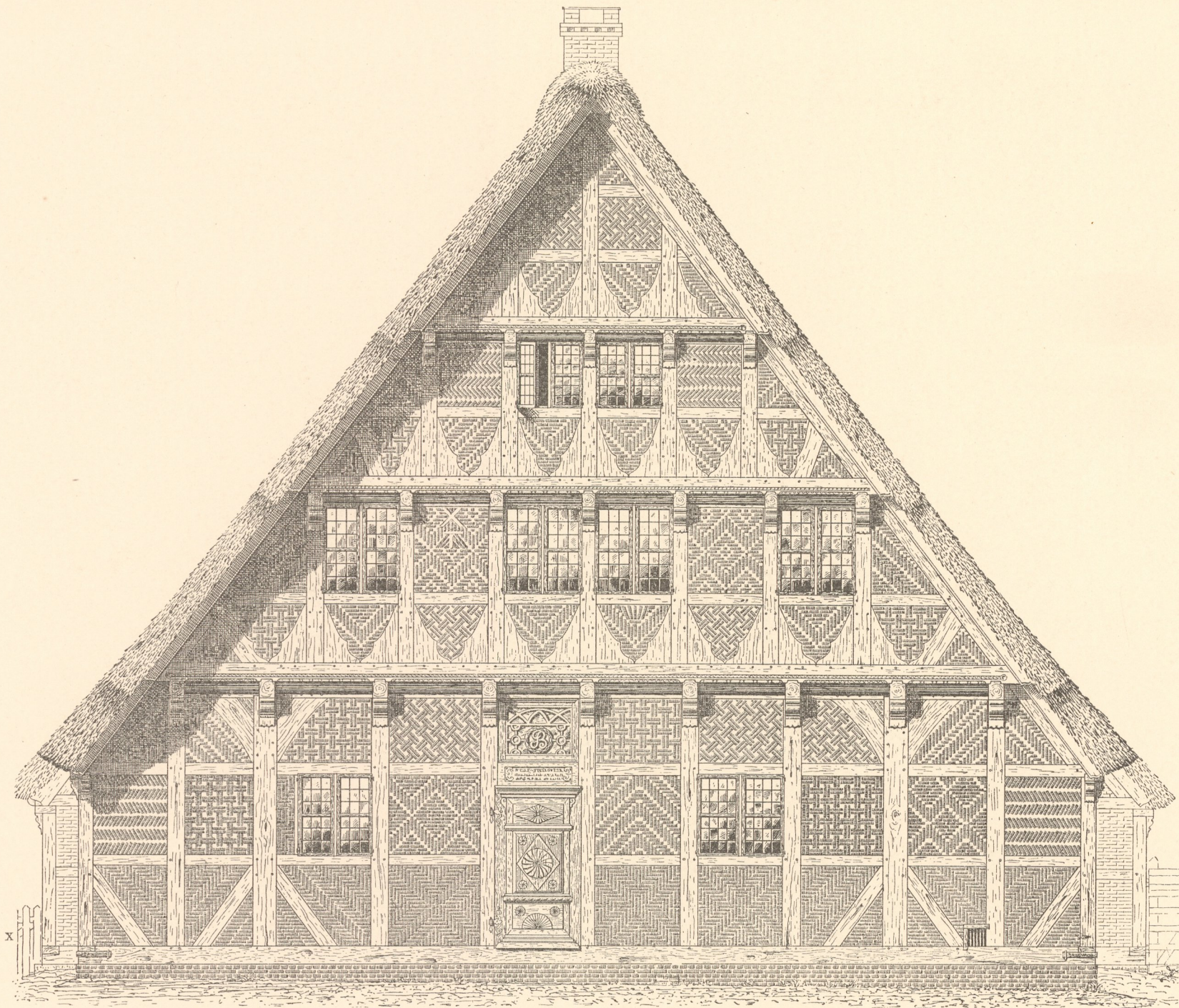
Abb. 1. Vorderansicht.
