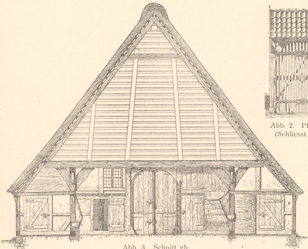
Abb. 3. Schnitt gh.
