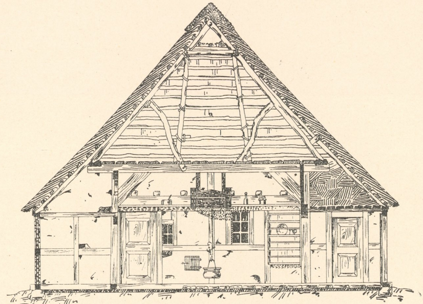
Abb. 5. Querschnitt a b.
