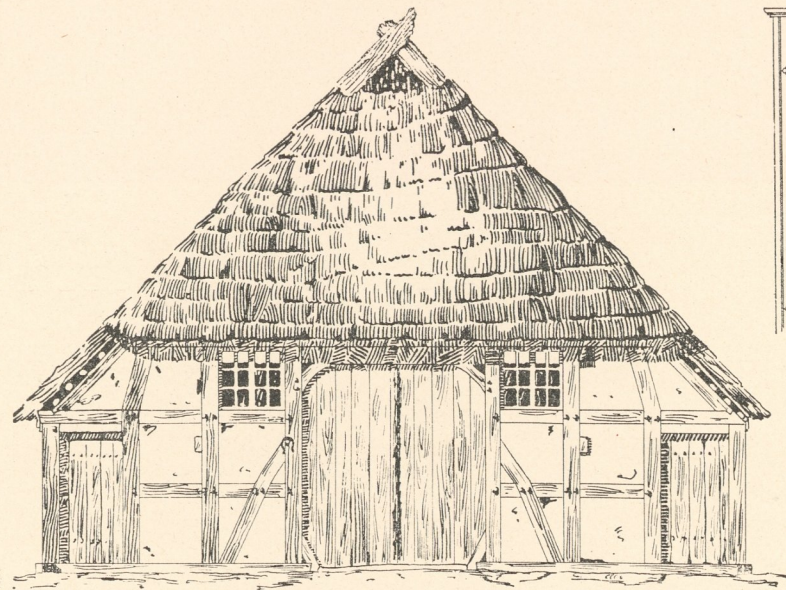
Abb. 4. Nordostansicht.
