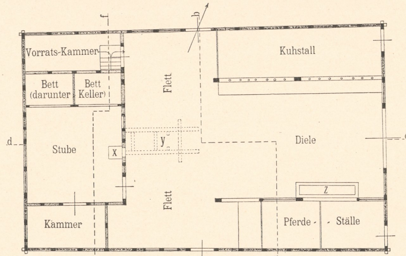
Abb. 1. Grundriss. x Ofen y Feuerstelle z Krippe.
