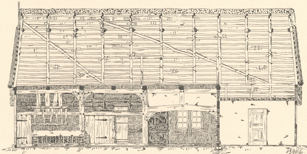
Abb. 6. Längenschnitt c d.
