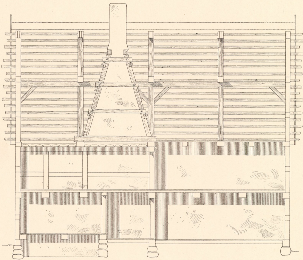
Abb. 2. Längenschnitt a b.
