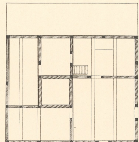
Abb. 6. Obergeschoss.
