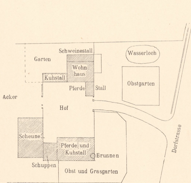
Abb. 4. Lageplan.
