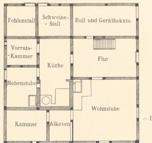
Abb. 5. Erdgeschoss.
