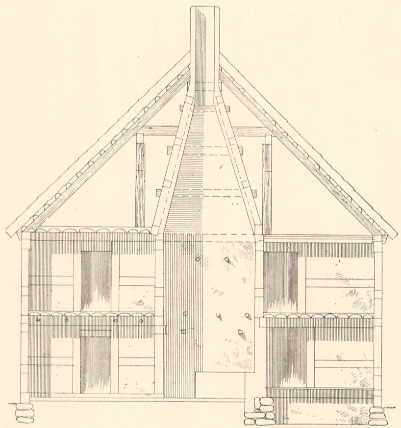
Abb. 3. Querschnitt c d.
