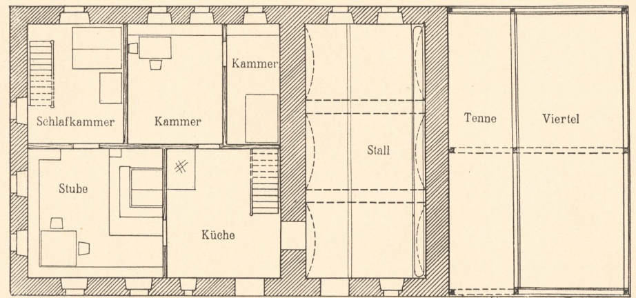
Abb. 6. Grundriss.
