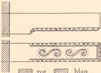
Abb. 8. Balkenkopf der Giebelaltane.
