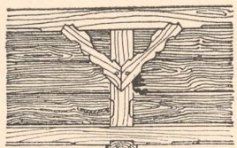
Abb. 7. Galeriedetail.
