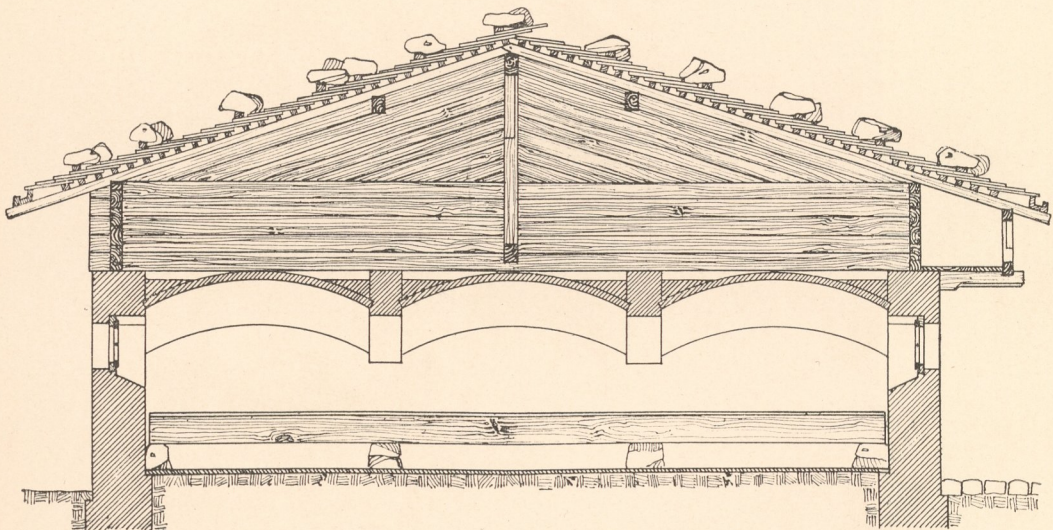
Abb. 4. Schnitt durch den Stall.
