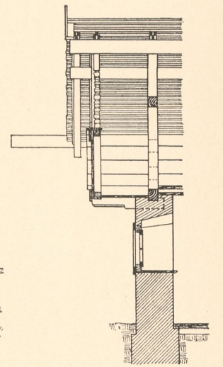
Abb. 5. Frontschnitt.
