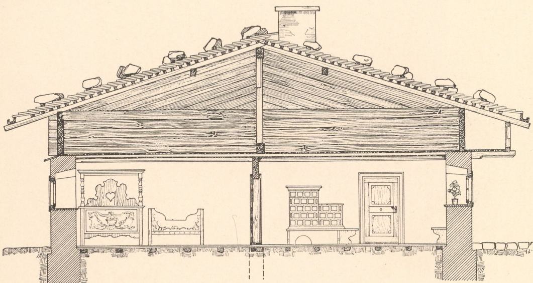
Abb. 2. Schnitt durch die Wohn- und Schlafstube.
