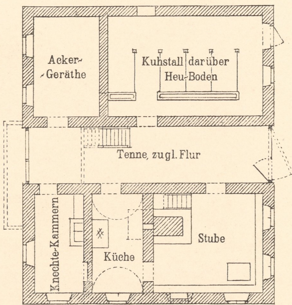
Abb. 1. Erdgeschoss.
