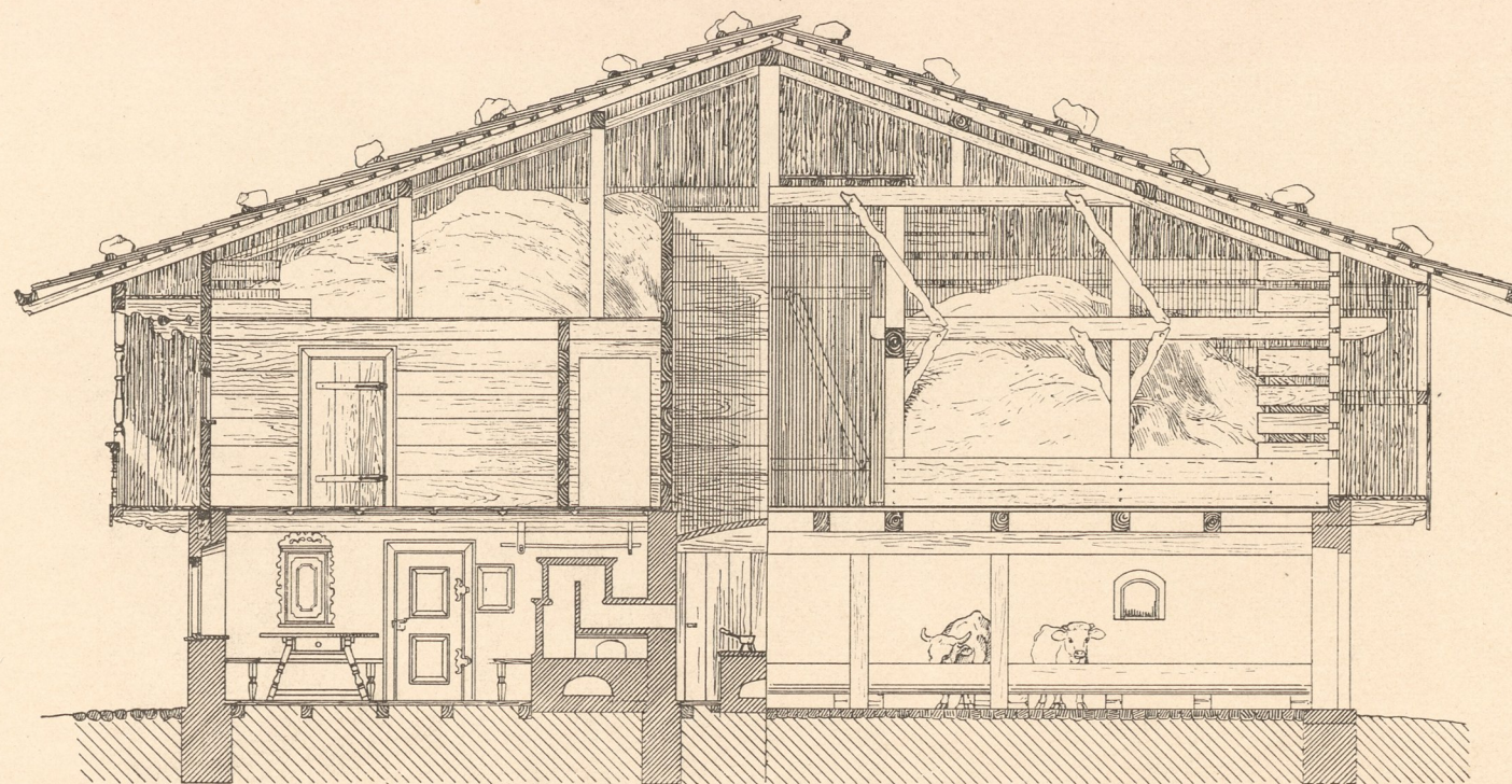
Abb. 2. Querschnitt A B.
