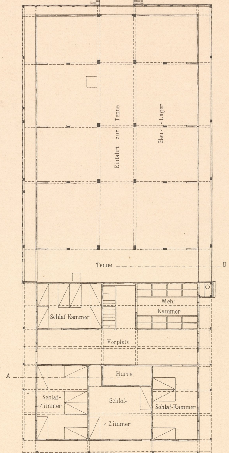
Abb. 4. Obergeschoss.
