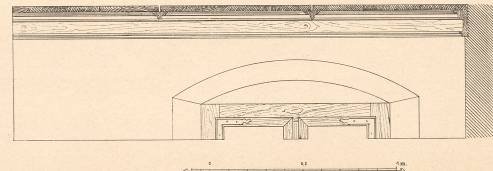
Abb. 7. Schnitt durch die Zimmerdecke (Schliersee).
