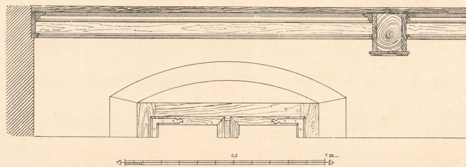
Abb. 5. Schnitt durch die Zimmerdecke (Schliersee).
