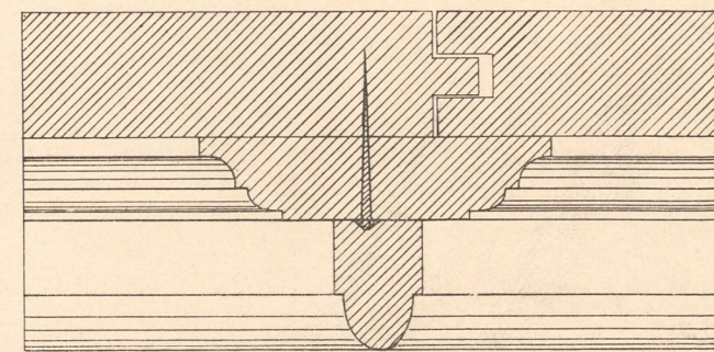
Abb. 6. Detail zur Zimmerdecke (Schliersee Bl. Bayern Nr. 7).
