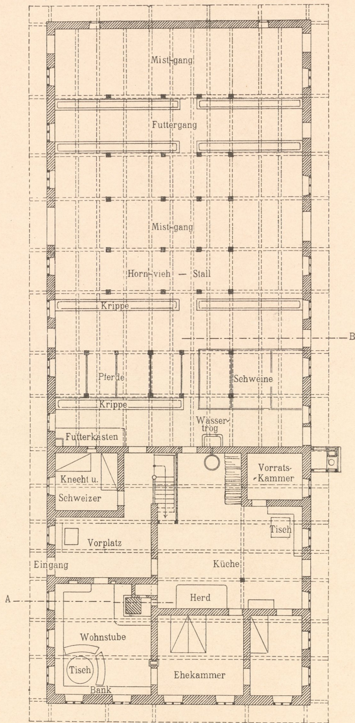
Abb. 3. Erdgeschoss.
