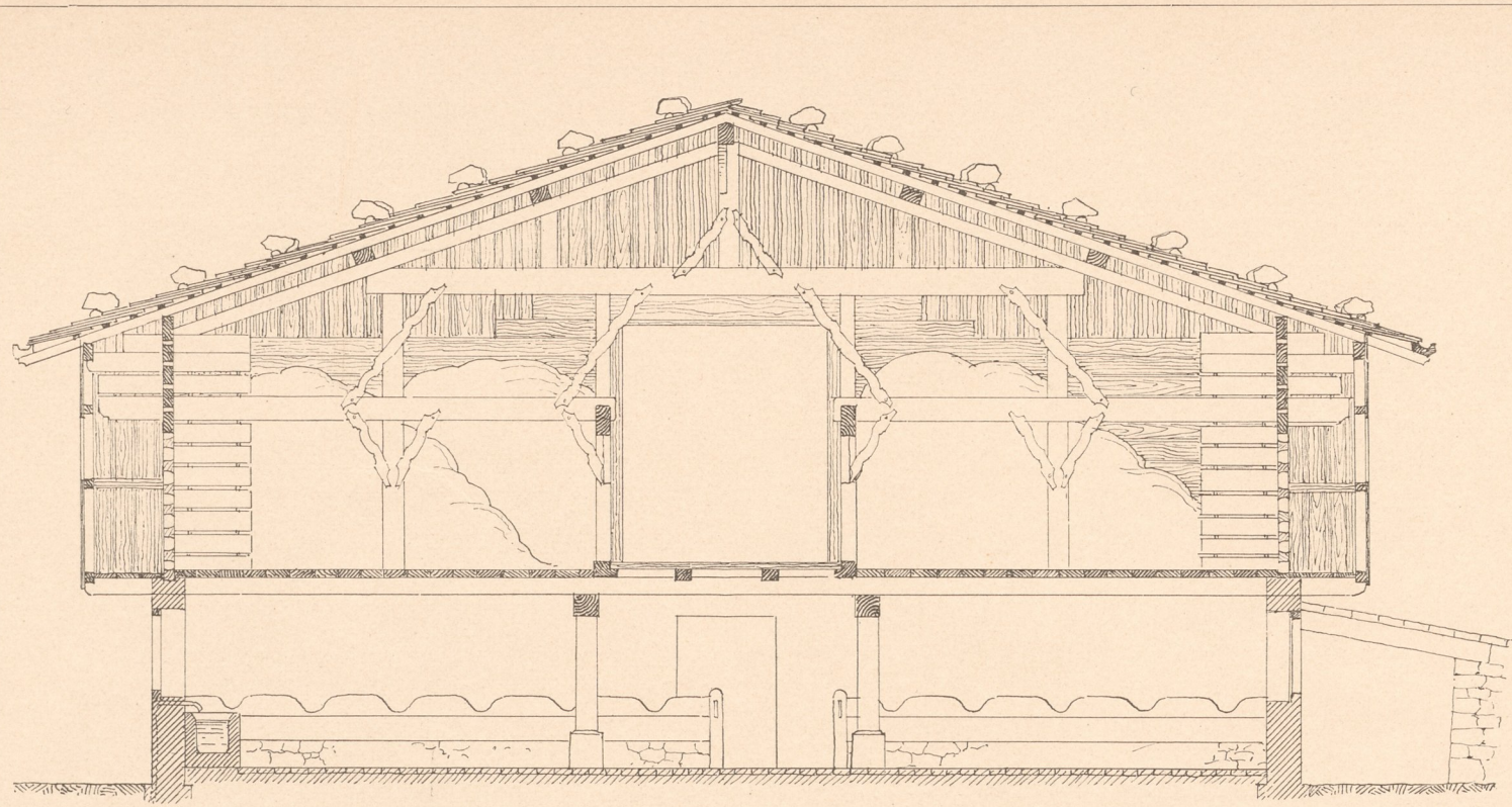
Abb. 2. Schnitt AB.
