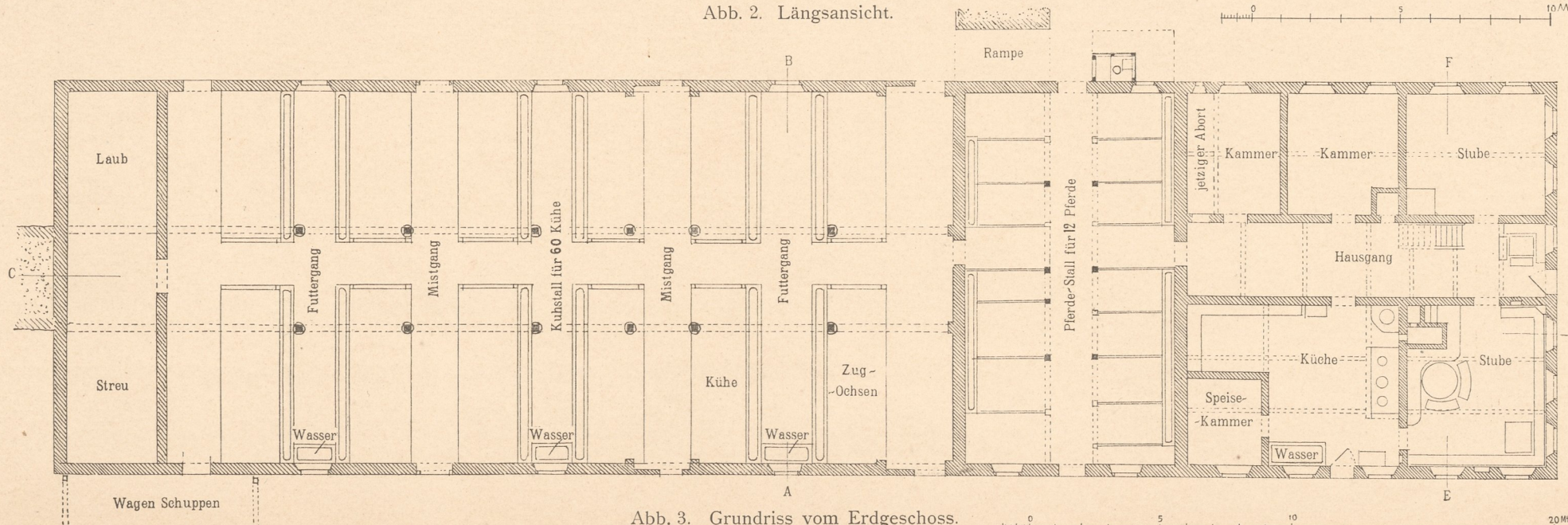
Abb. 3. Grundriss vom Erdgeschoss.
