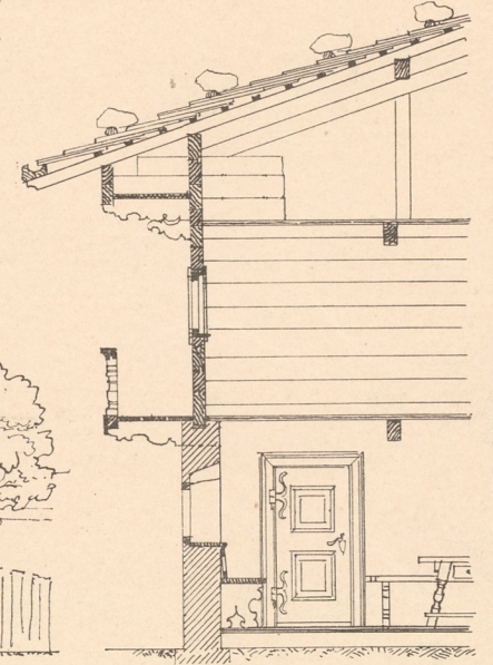
Abb. 5. Schnitt bei E.
