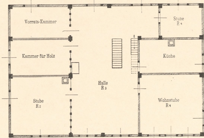
Abb. 5. Grundriss des Obergeschosses.
