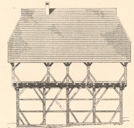
Abb. 9. Längsansicht. Ursprünglicher Zustand.
