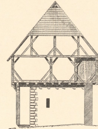
Abb. 8. Giebelansicht. Ursprünglicher Zustand.
