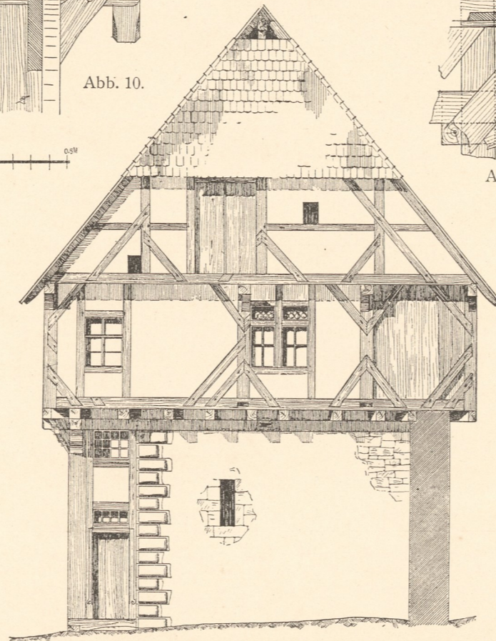
Abb. 4. Giebelansicht.
