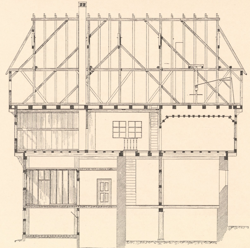
Abb. 3. Längsschnitt C D.
